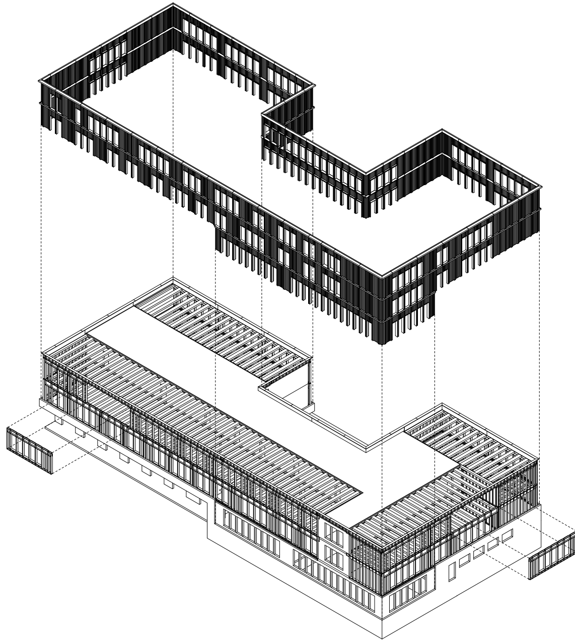
Neubau Heilpädagogische Schule Lyss Axonometrie Konstruktiver Holzbau und Fassade
