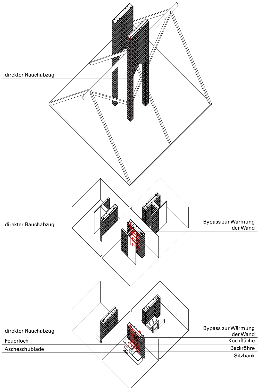
Feuerungsanlage mit Rauchabzug
