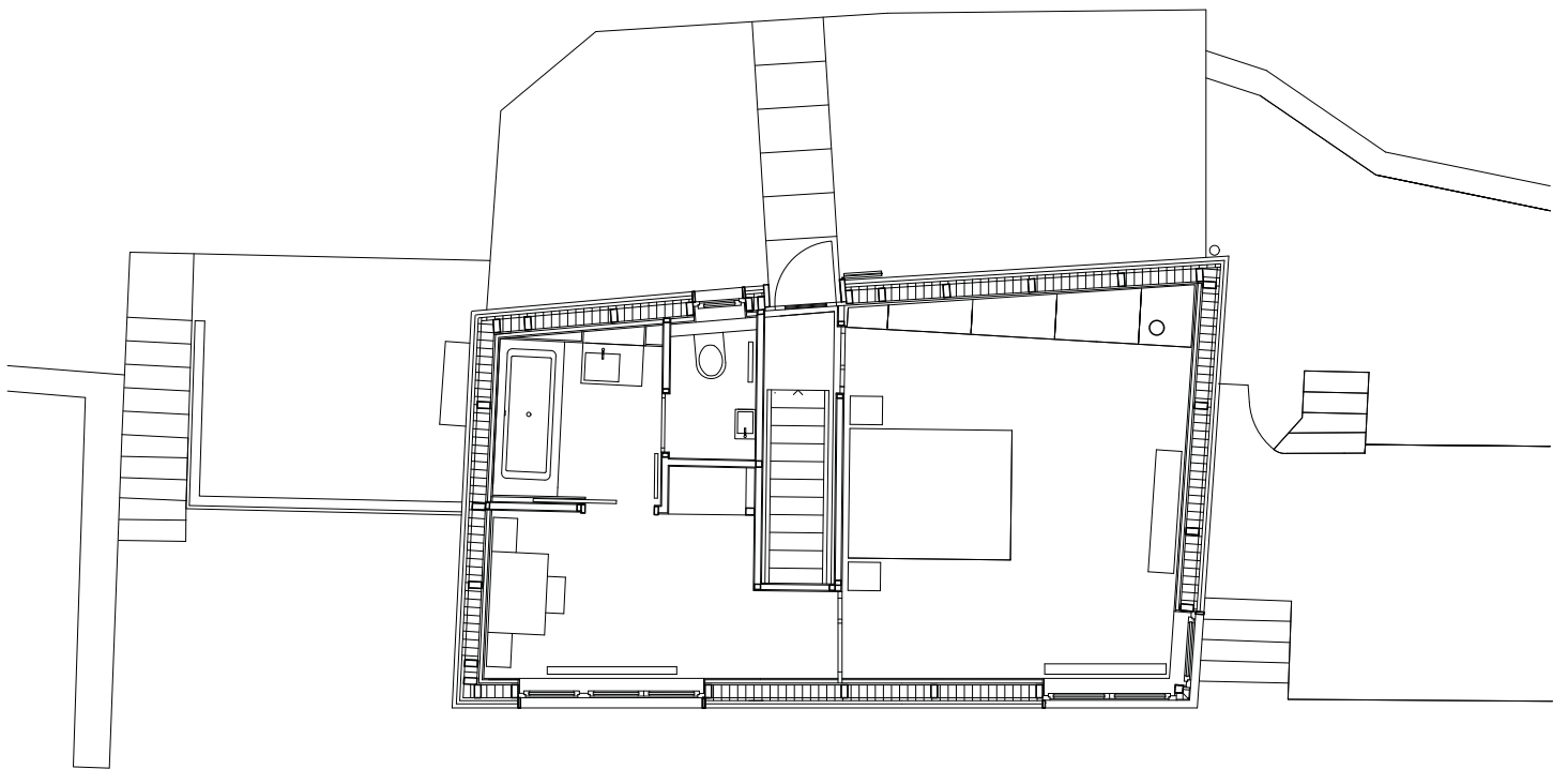
Grundriss 2. Obergeschoss
