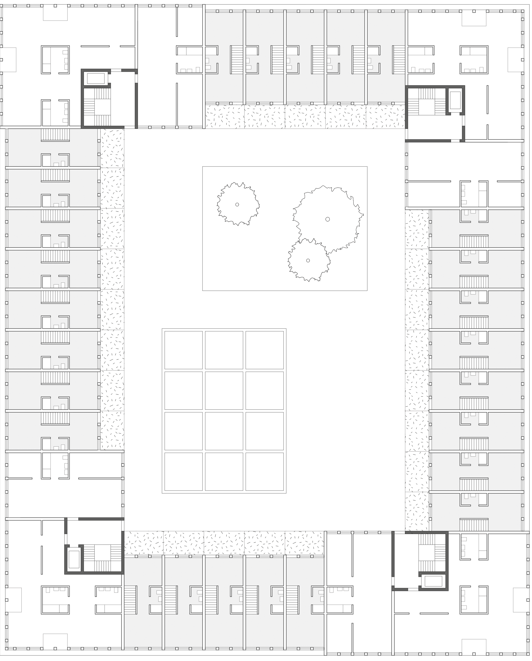
GRUNDRISS WOHNEN 1:200
