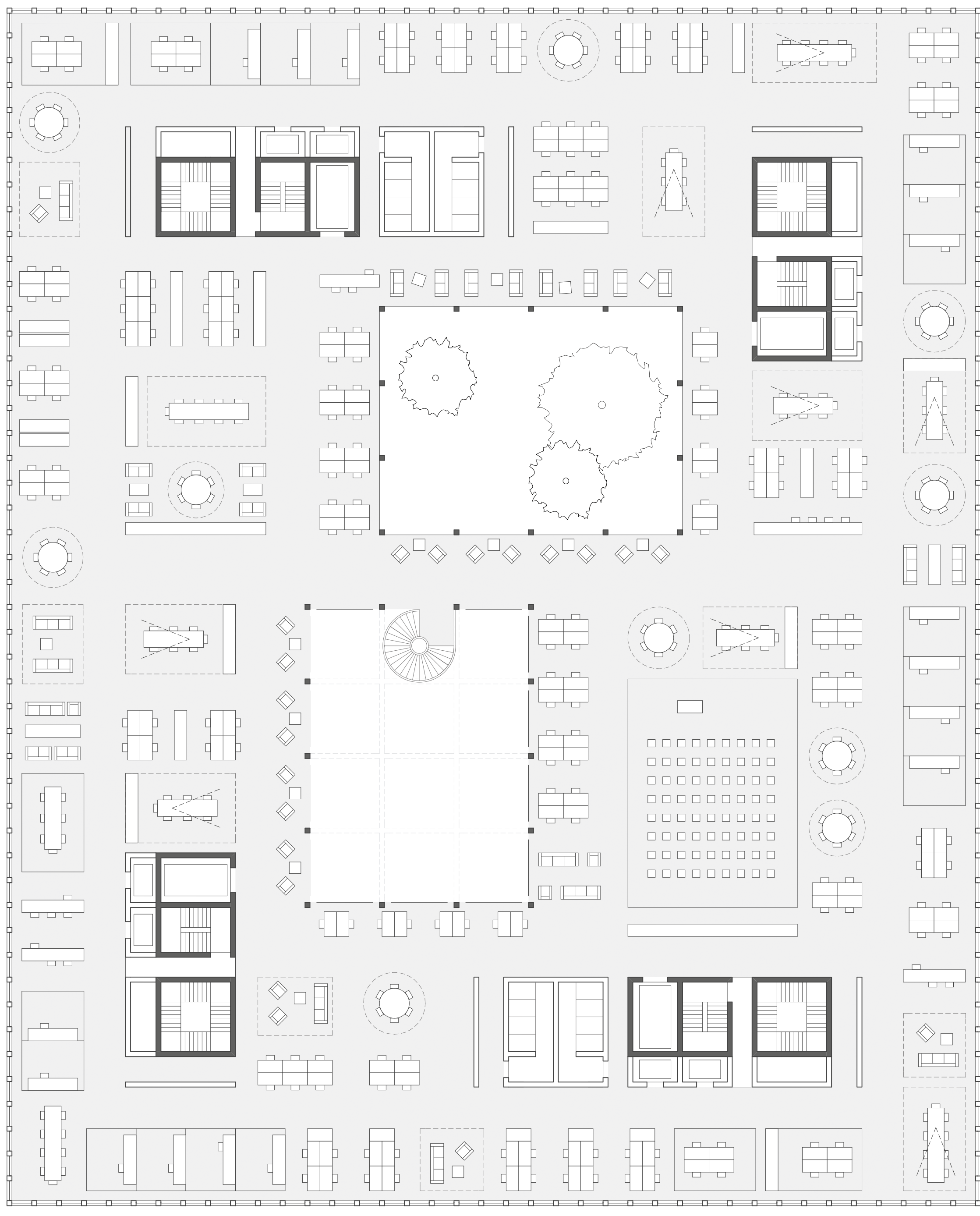
GRUNDRISS ARBEITEN 1:200
