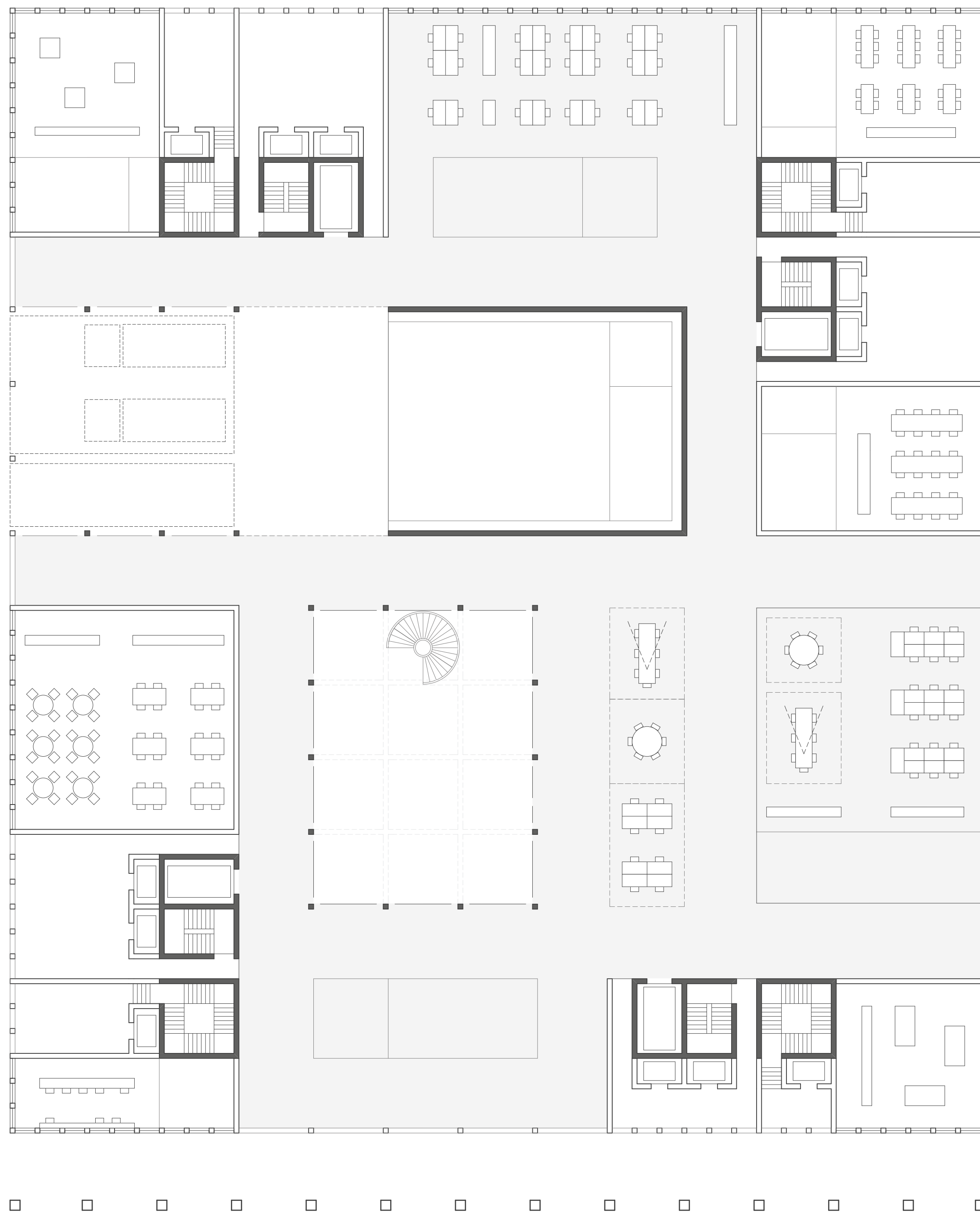
GRUNDRISS ERDGESCHOSS 1:200
