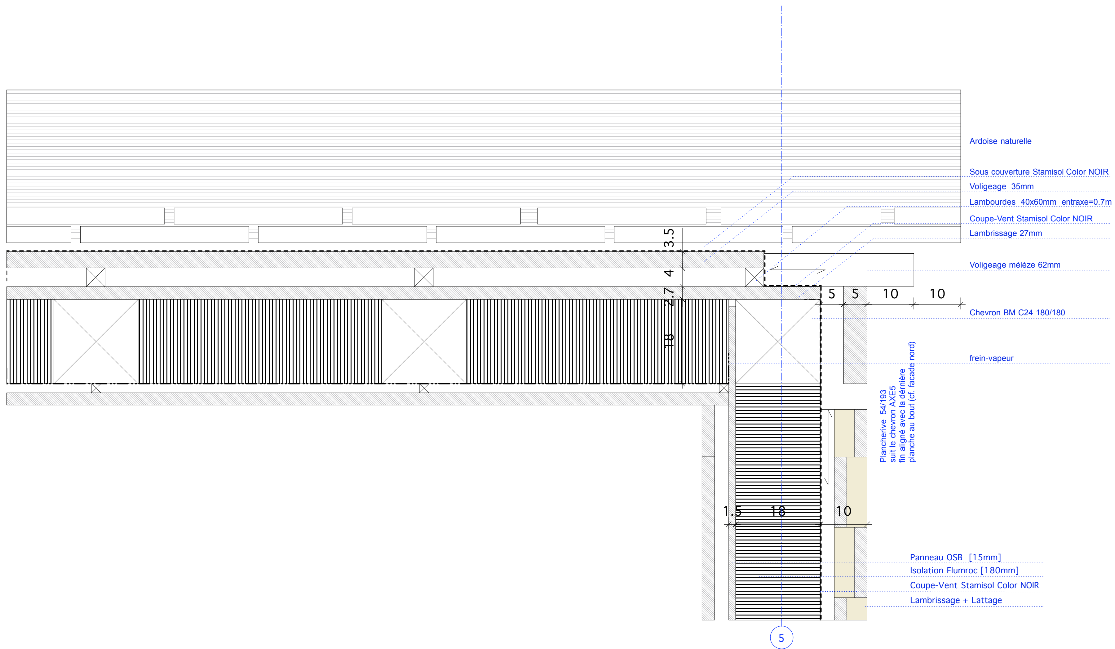
détail pignon
