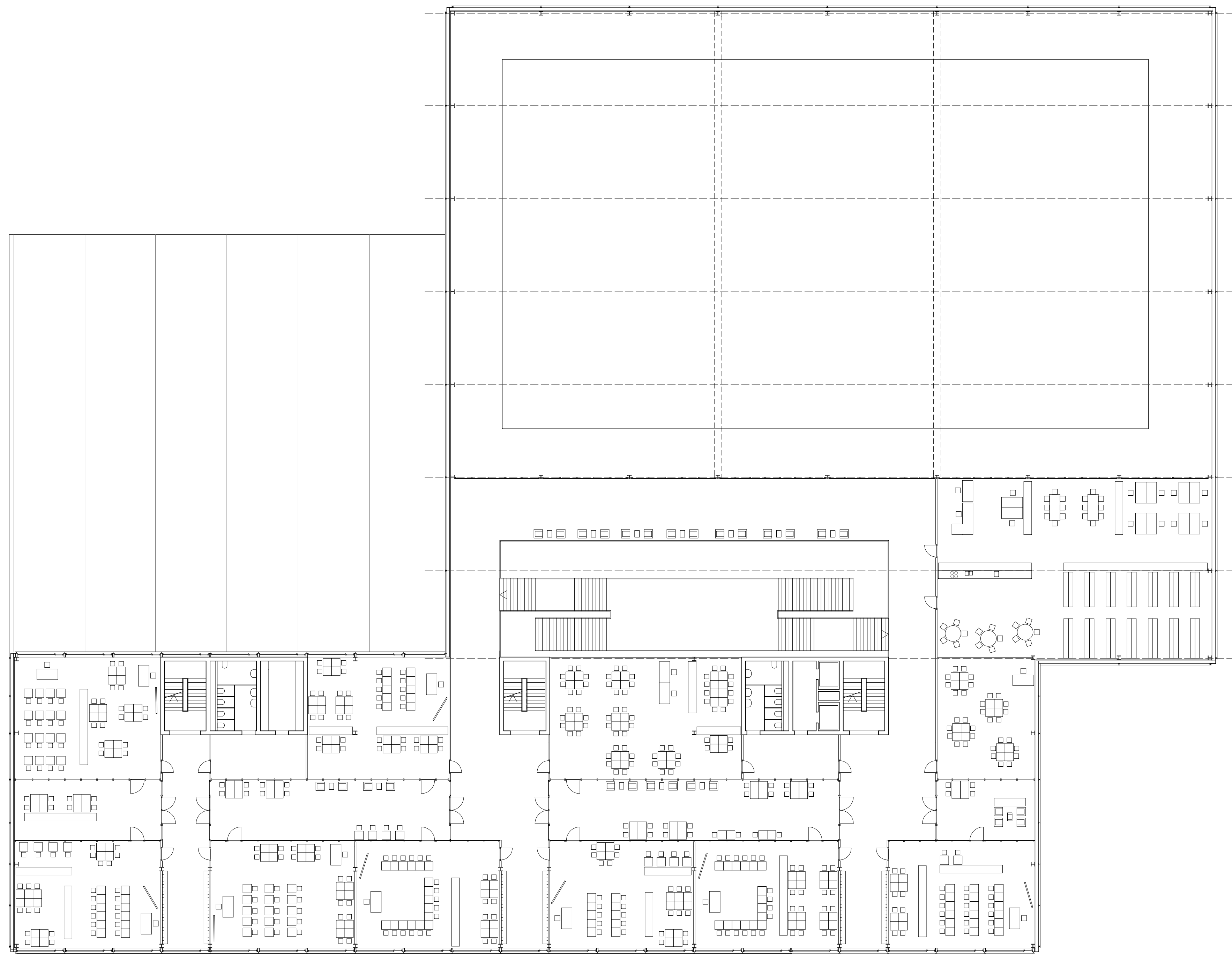
2. Obergeschoss 1:200
