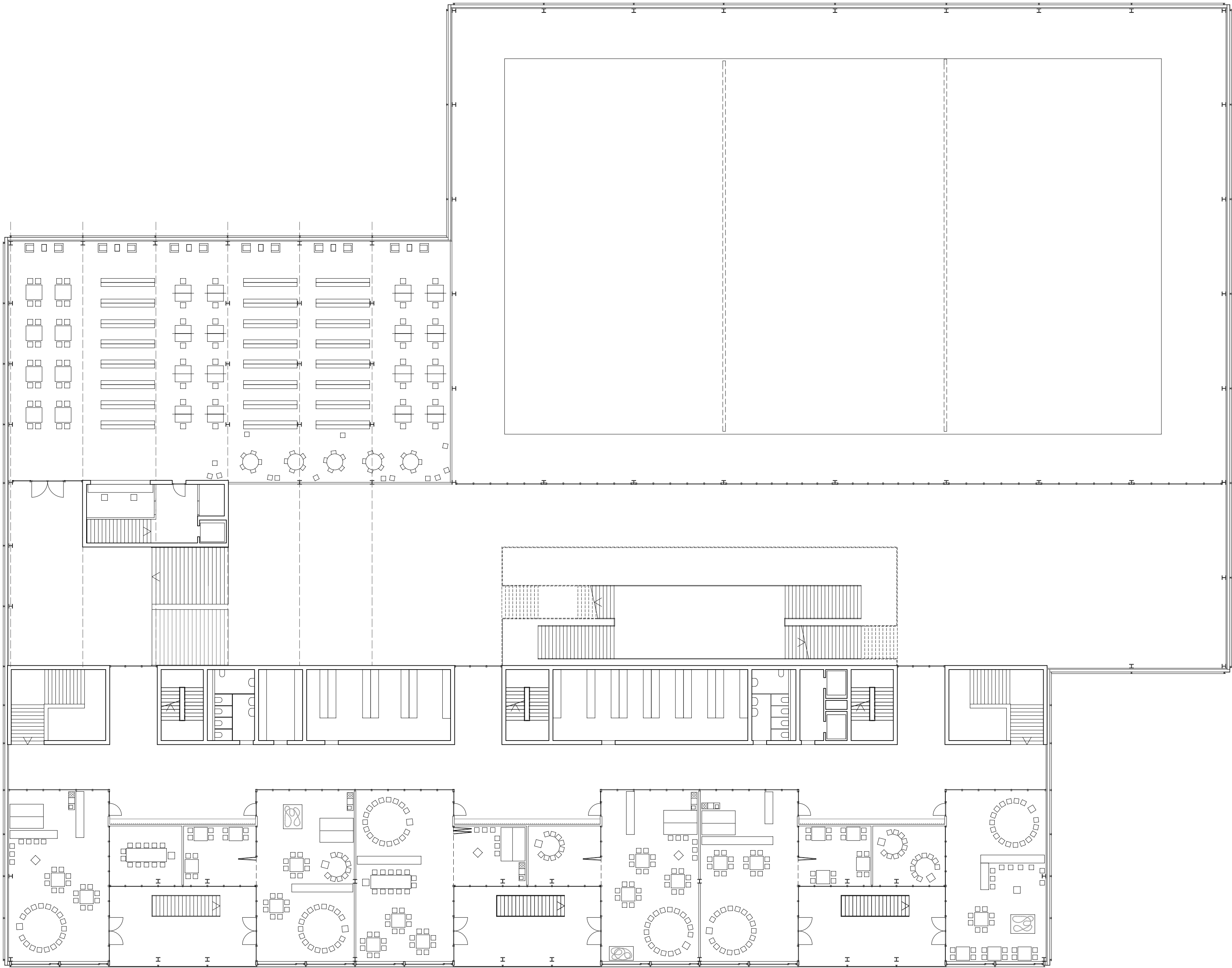
1. Obergeschoss 1:200
