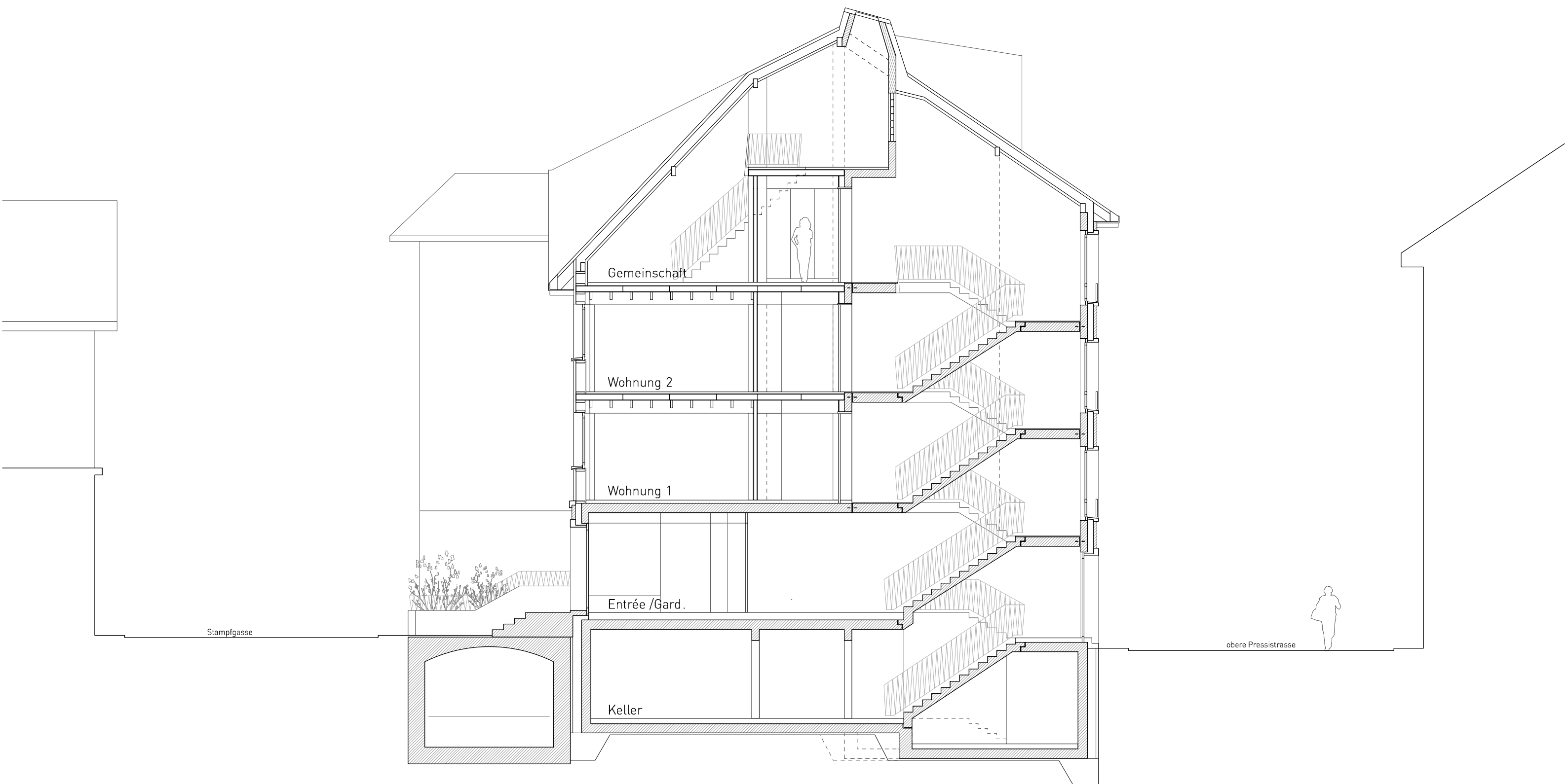
Schnitt B 1_100
