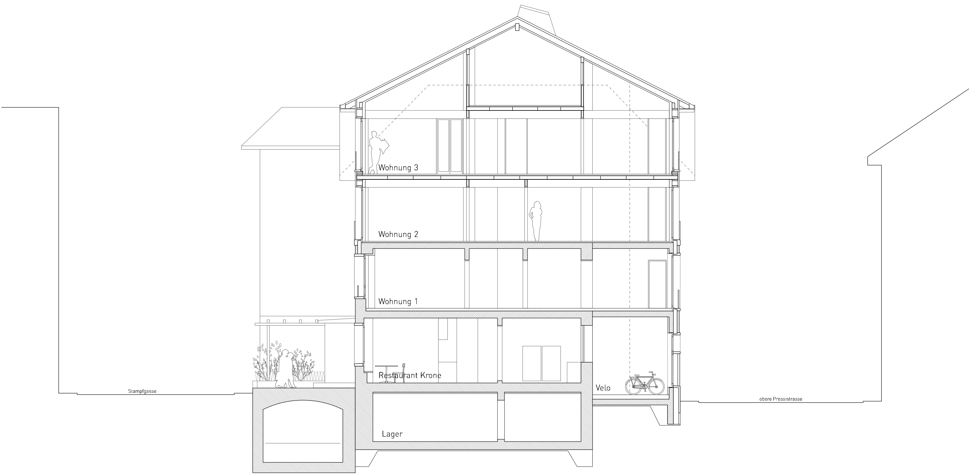
Schnitt C 1_100
