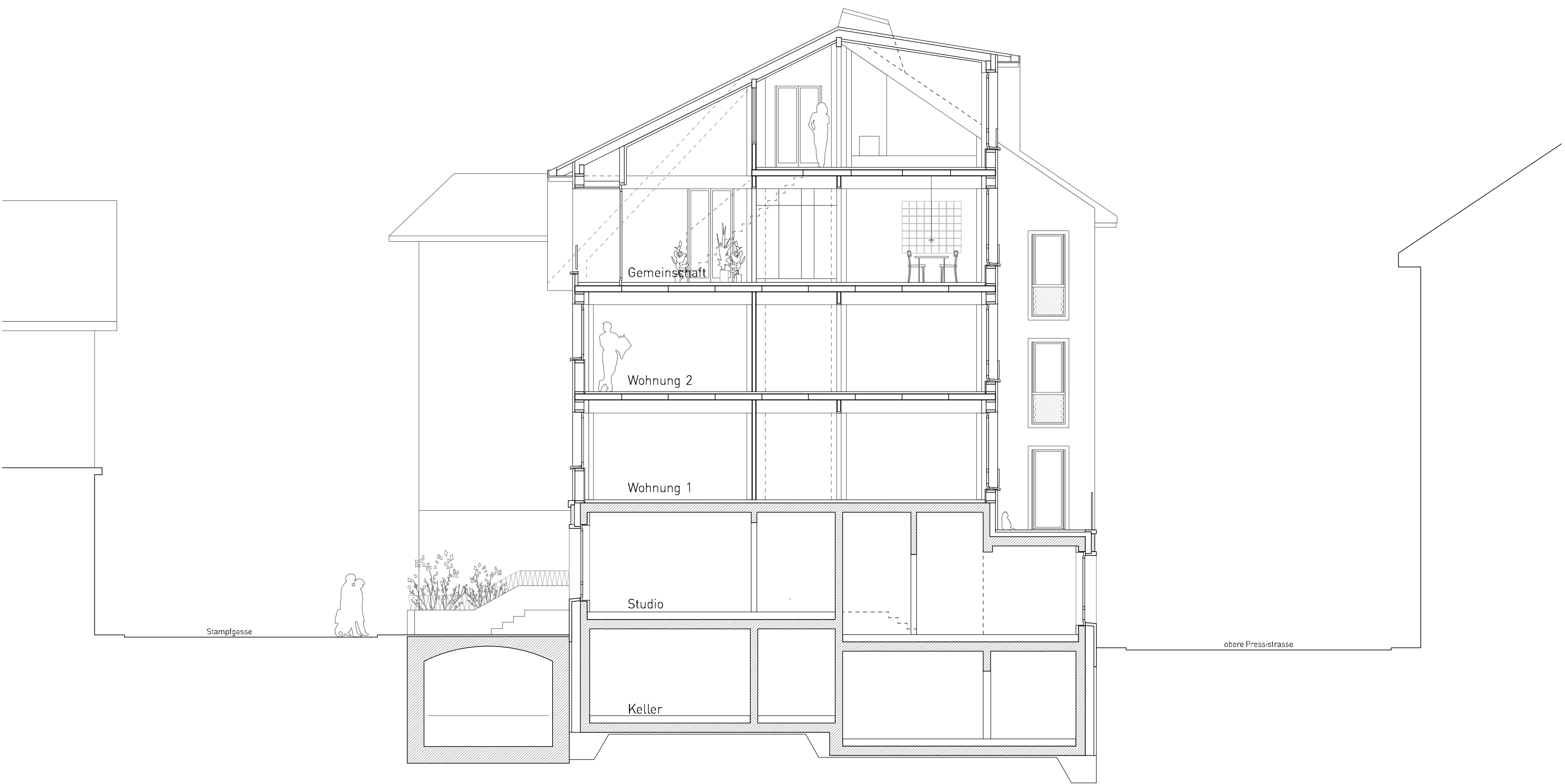
Schnitt A 1_100
