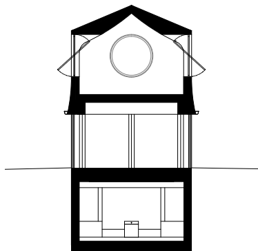
Schnitt A | Coupe A
