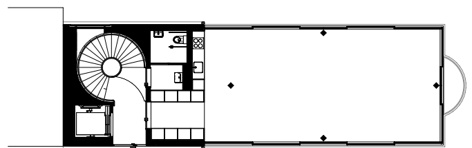
Erdgeschoss | Rez-de-chaussée
