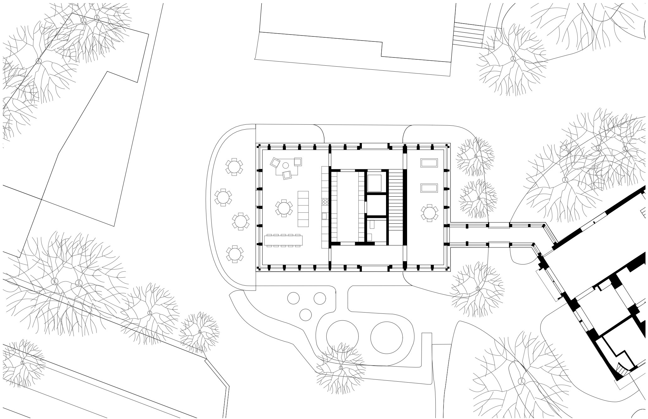
Erdgeschoss 1:200
