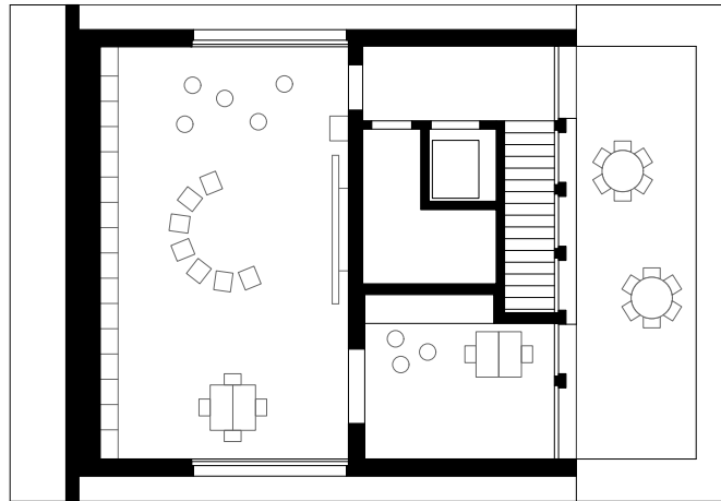
Dachgeschoss 1:200
