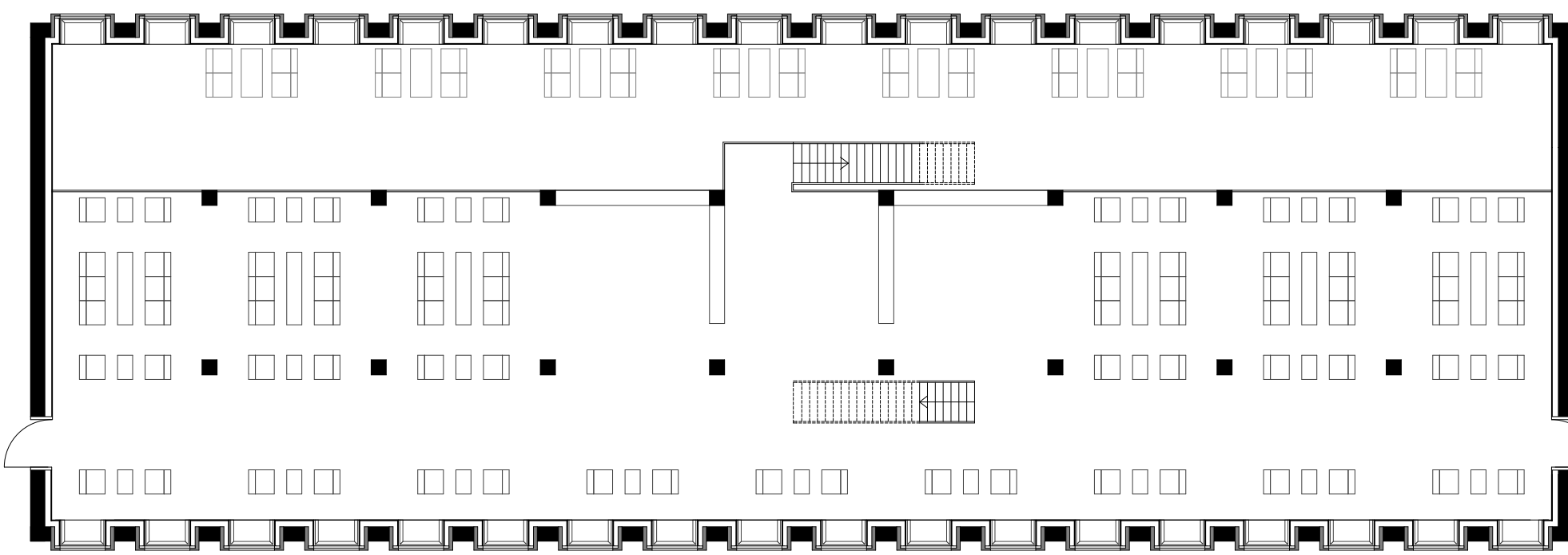
Kaffee-Stube 3, Obergeschoss | Mst.: 1:200
