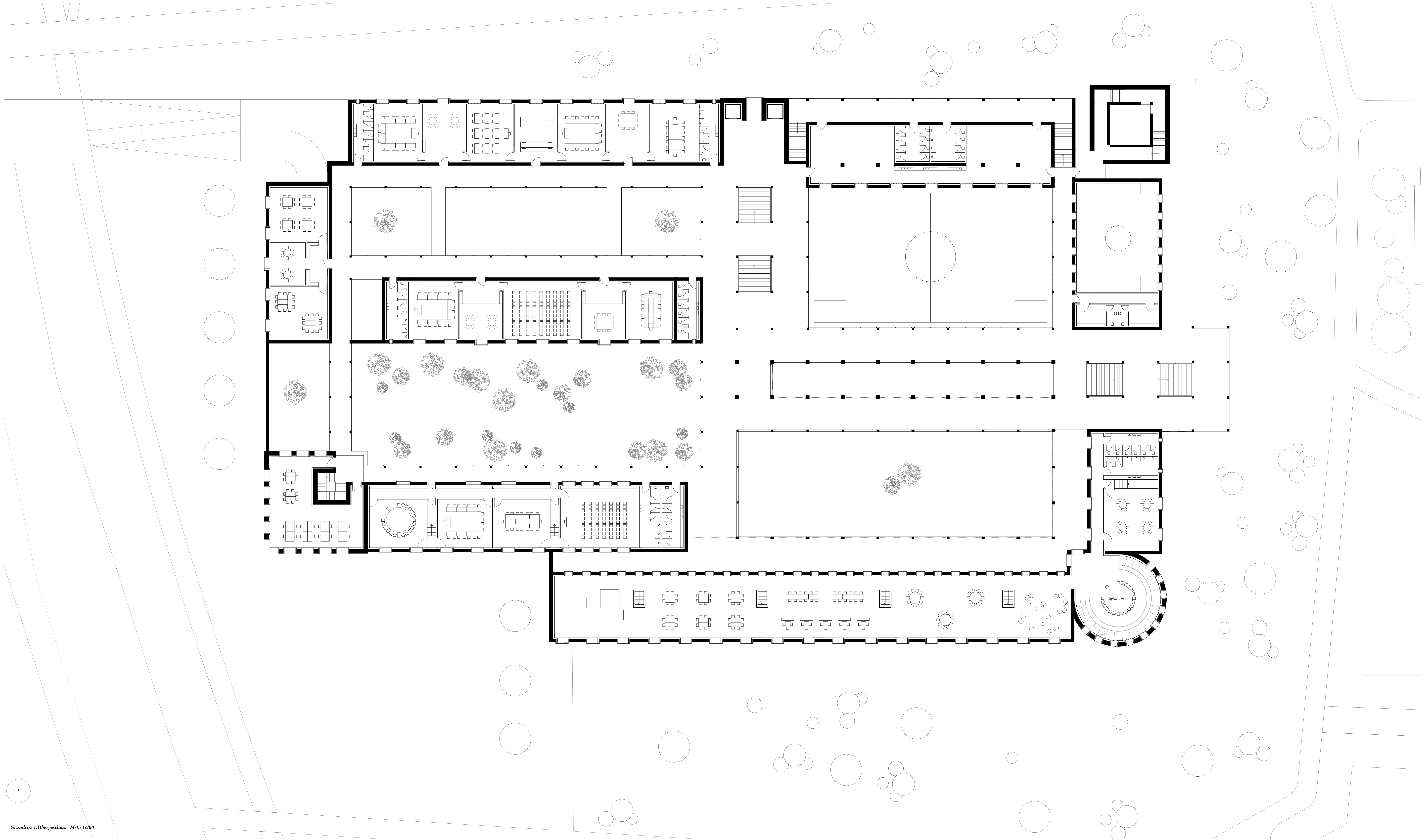
Mensa 2, Obergeschoss | Mst.: 1:200
