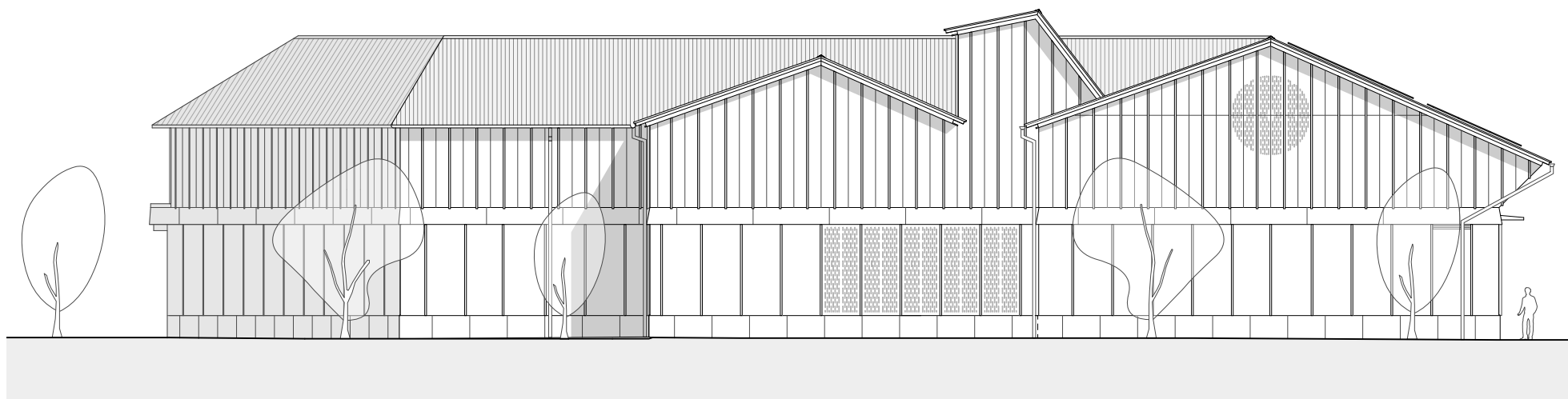
Ansicht Nord-West
