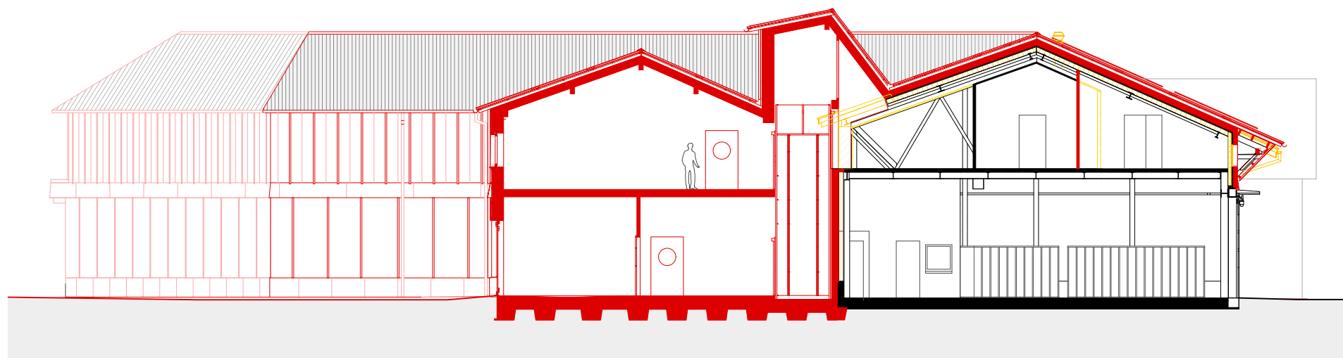
Schnitt AA
