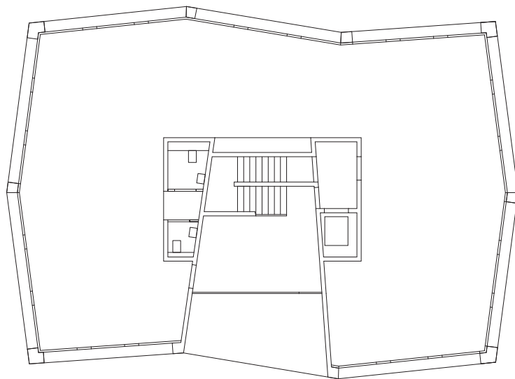
Rez-de-chaussée / 1:250 ème
