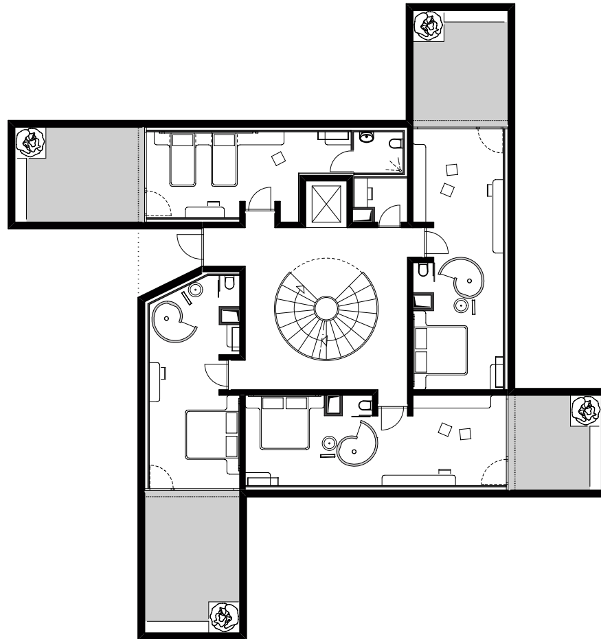
Pianta piano terreno
