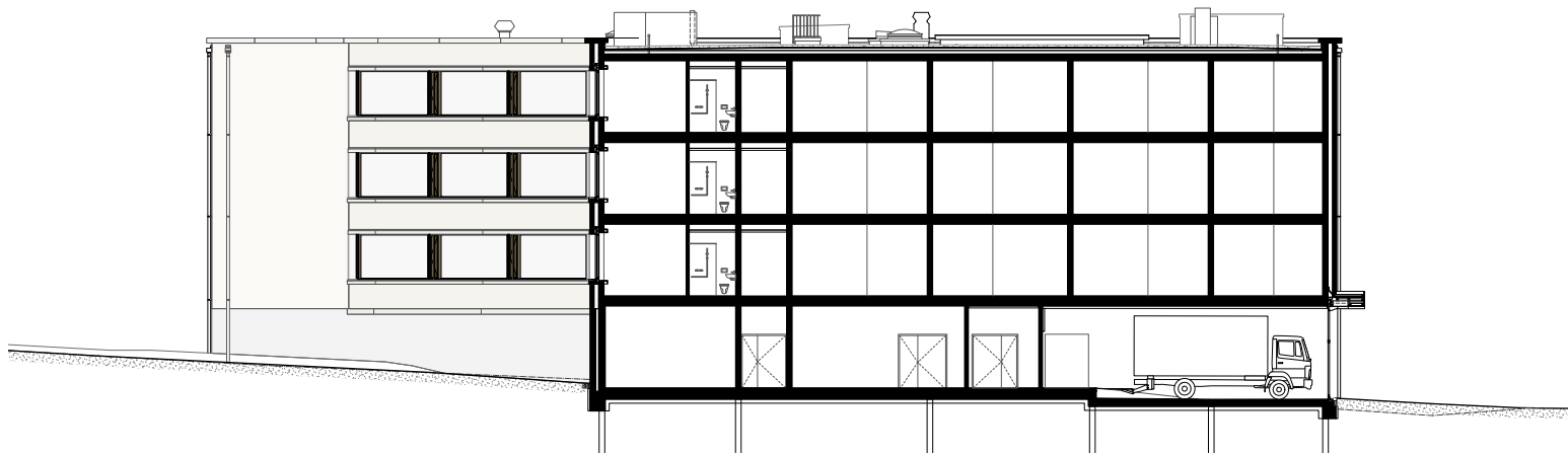
SCHNITT A-A
