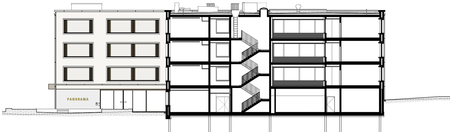
SCHNITT B-B
