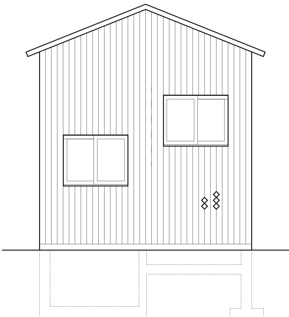
façade est 1:50
