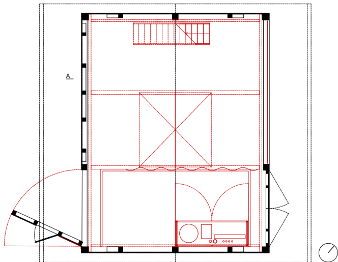
Erdgeschoss | Rez-de-chaussée
