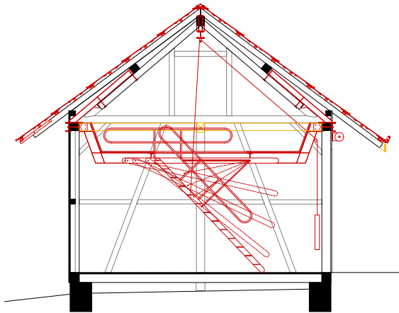
Schnitt A | Coupe A
