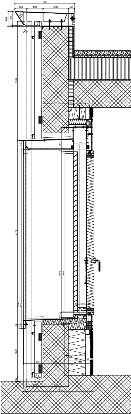
DETAIL PROTOTYPE COUPE 1:25
