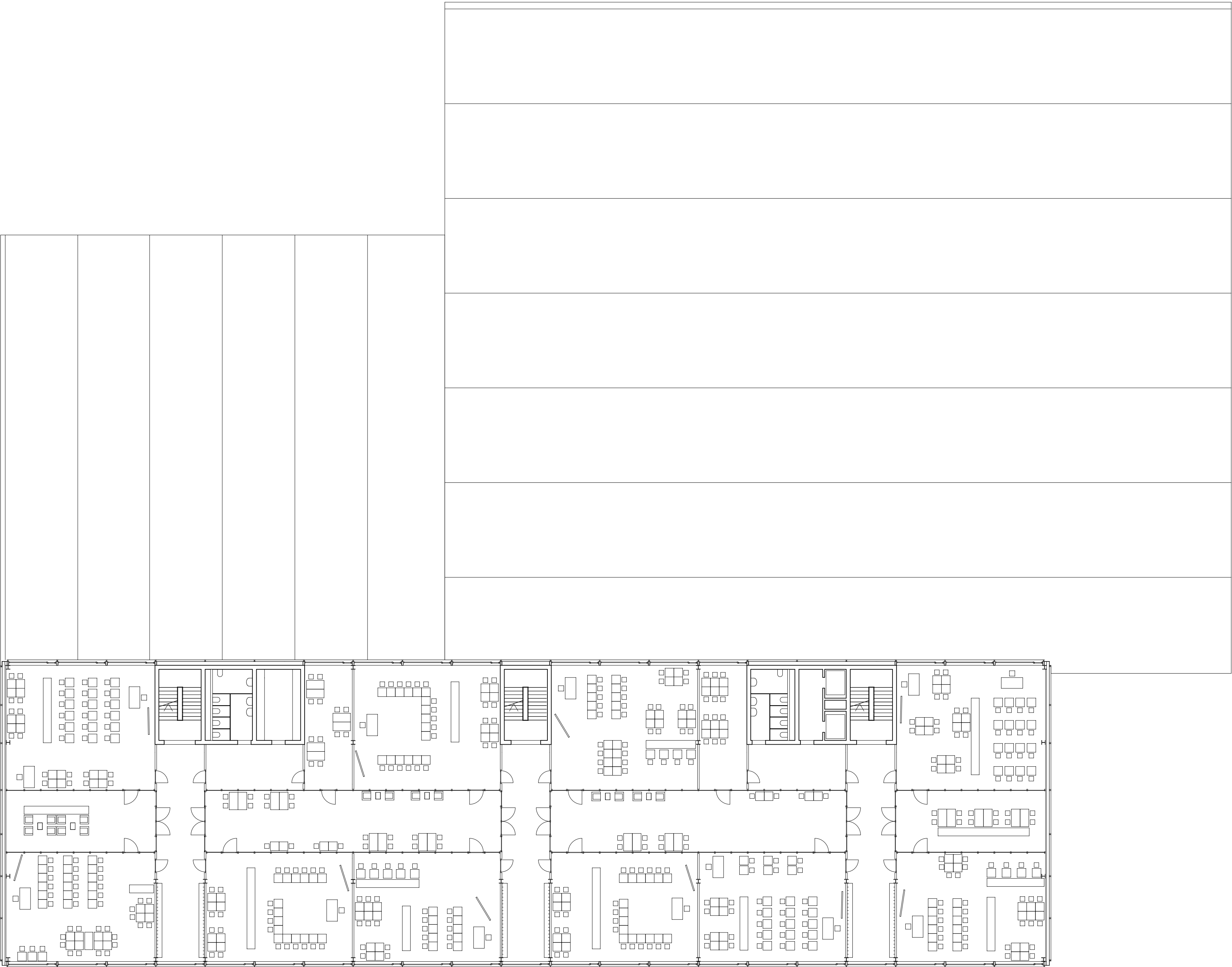
3.Obergeschoss 1:200
