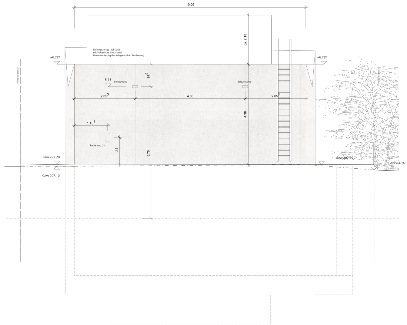
Ansicht - Ost
