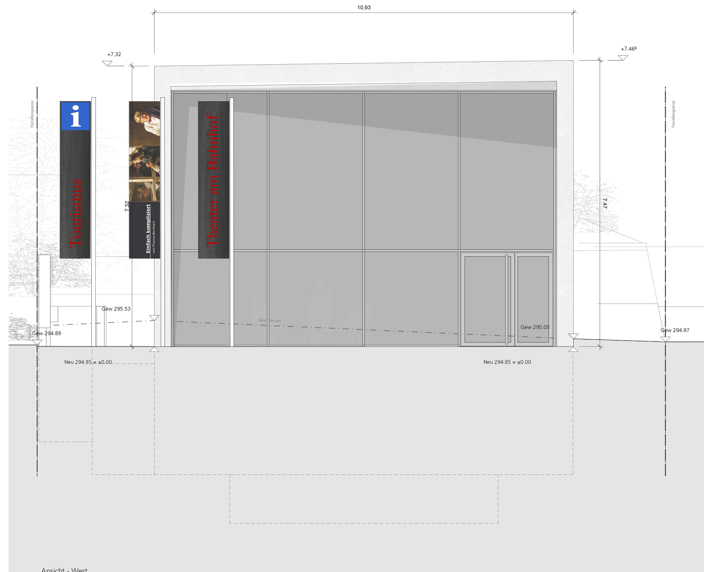
Ansicht - West
