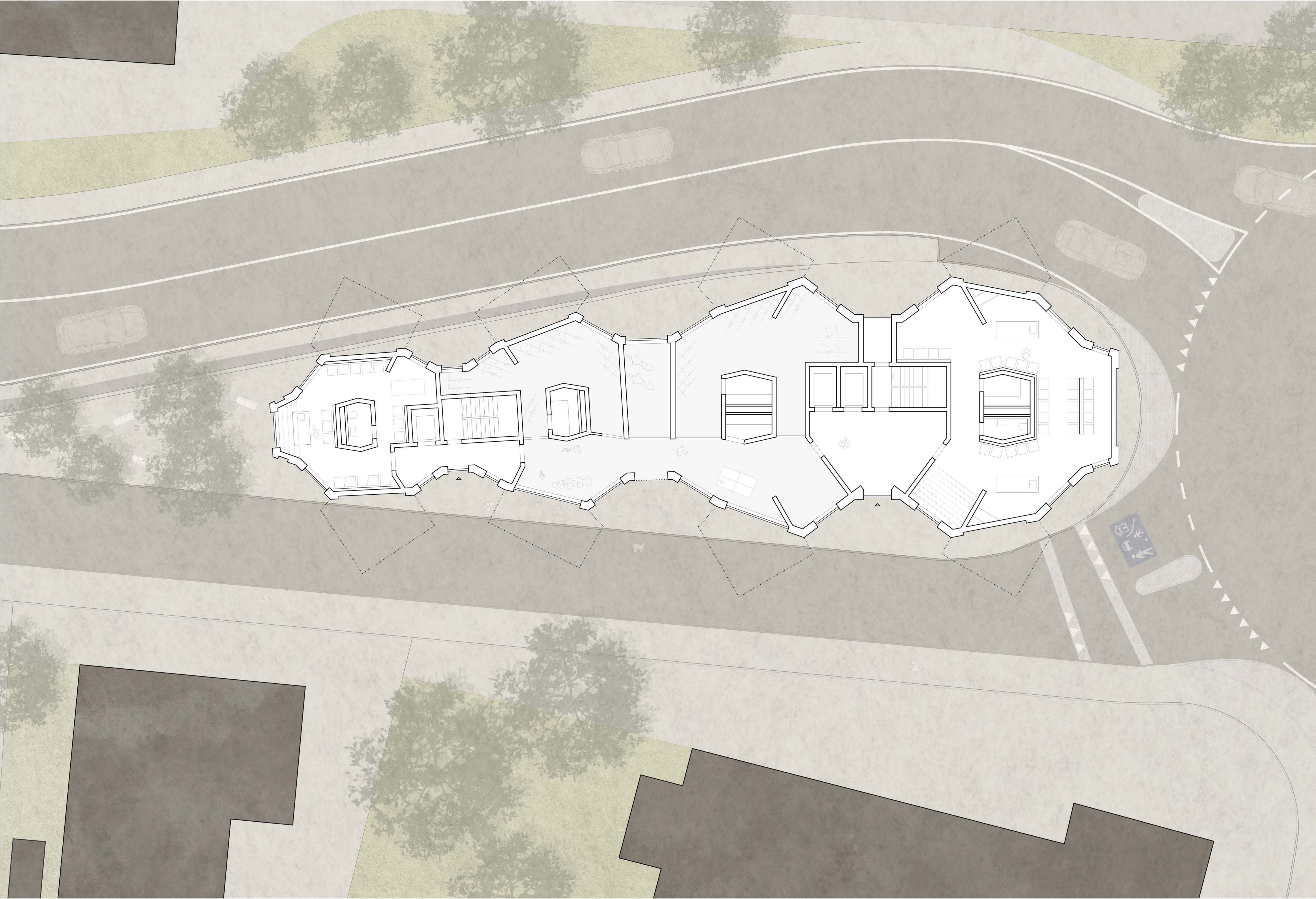
Erdgeschoss mit Umgebung | 1:100
