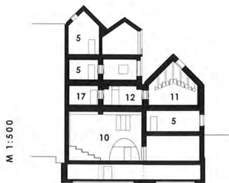
Querschnitt
