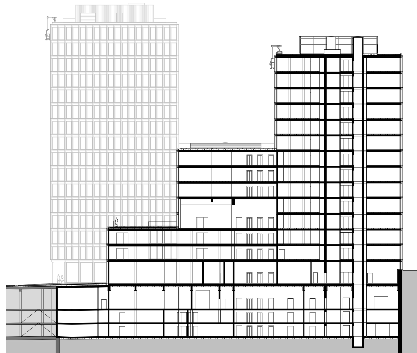
Coupe A-A
