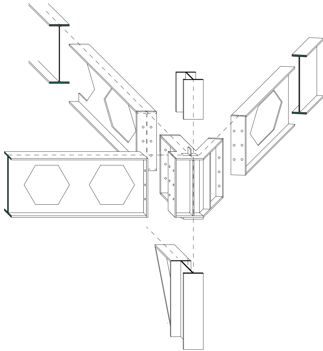
KONSTRUKTIONSDetail 1:33
