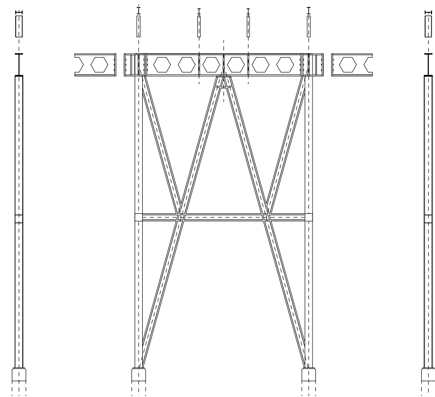
KONSTRUKTIONSSchema 1:150
