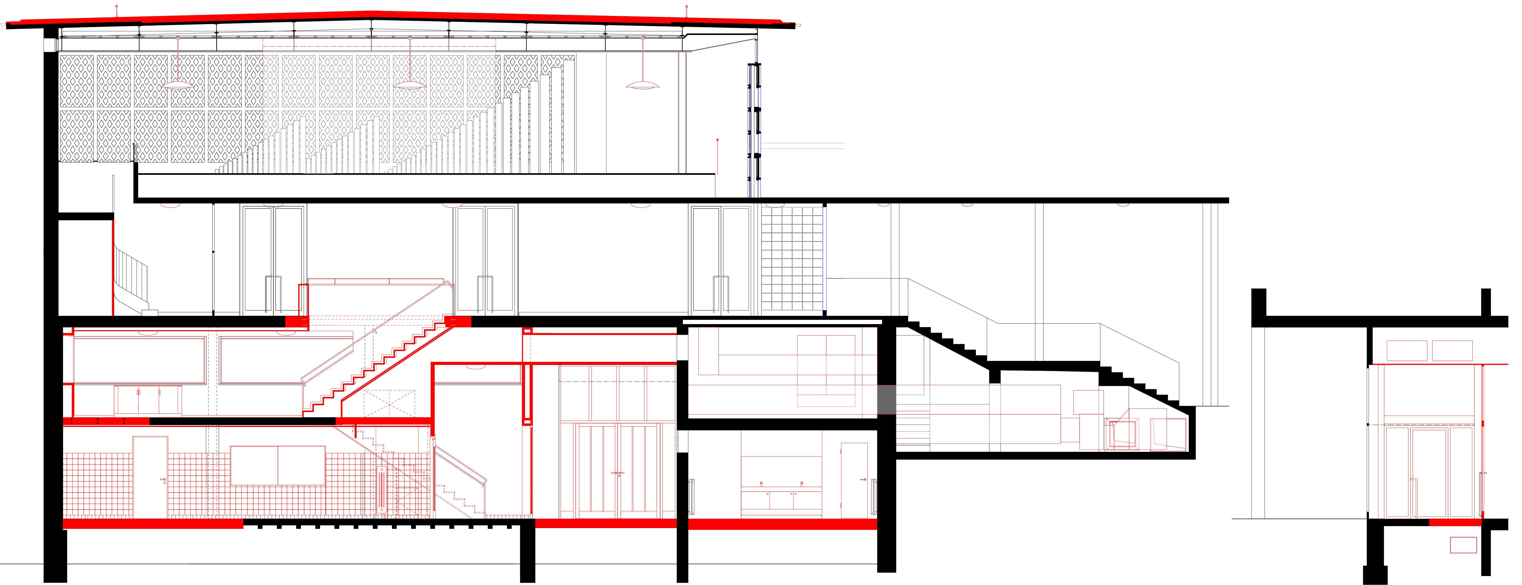
SCHNITT E-E
