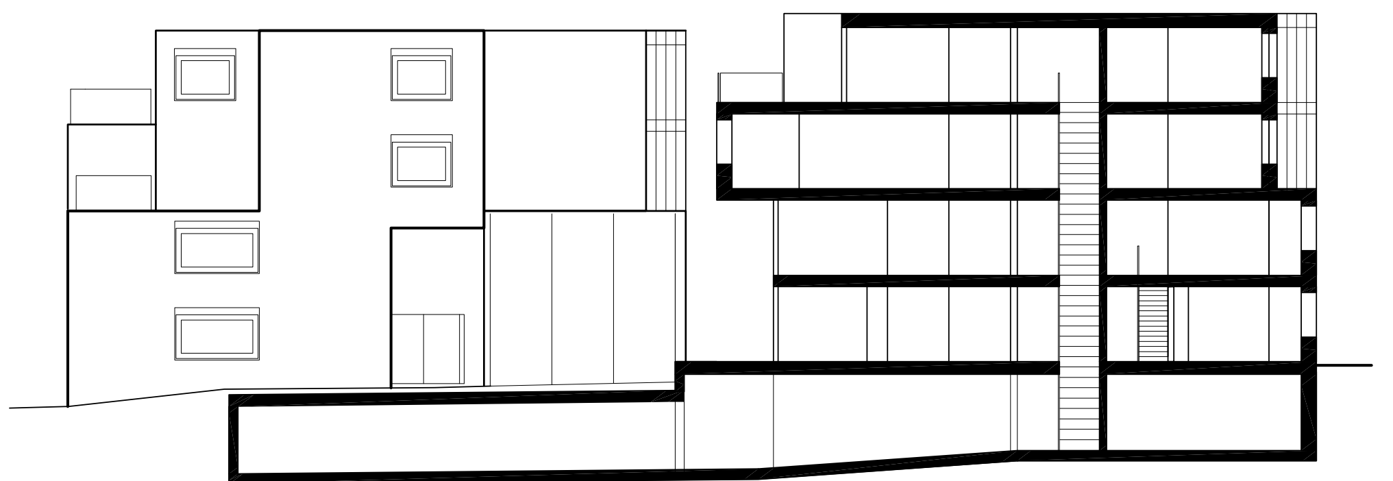
Coupe transversale
