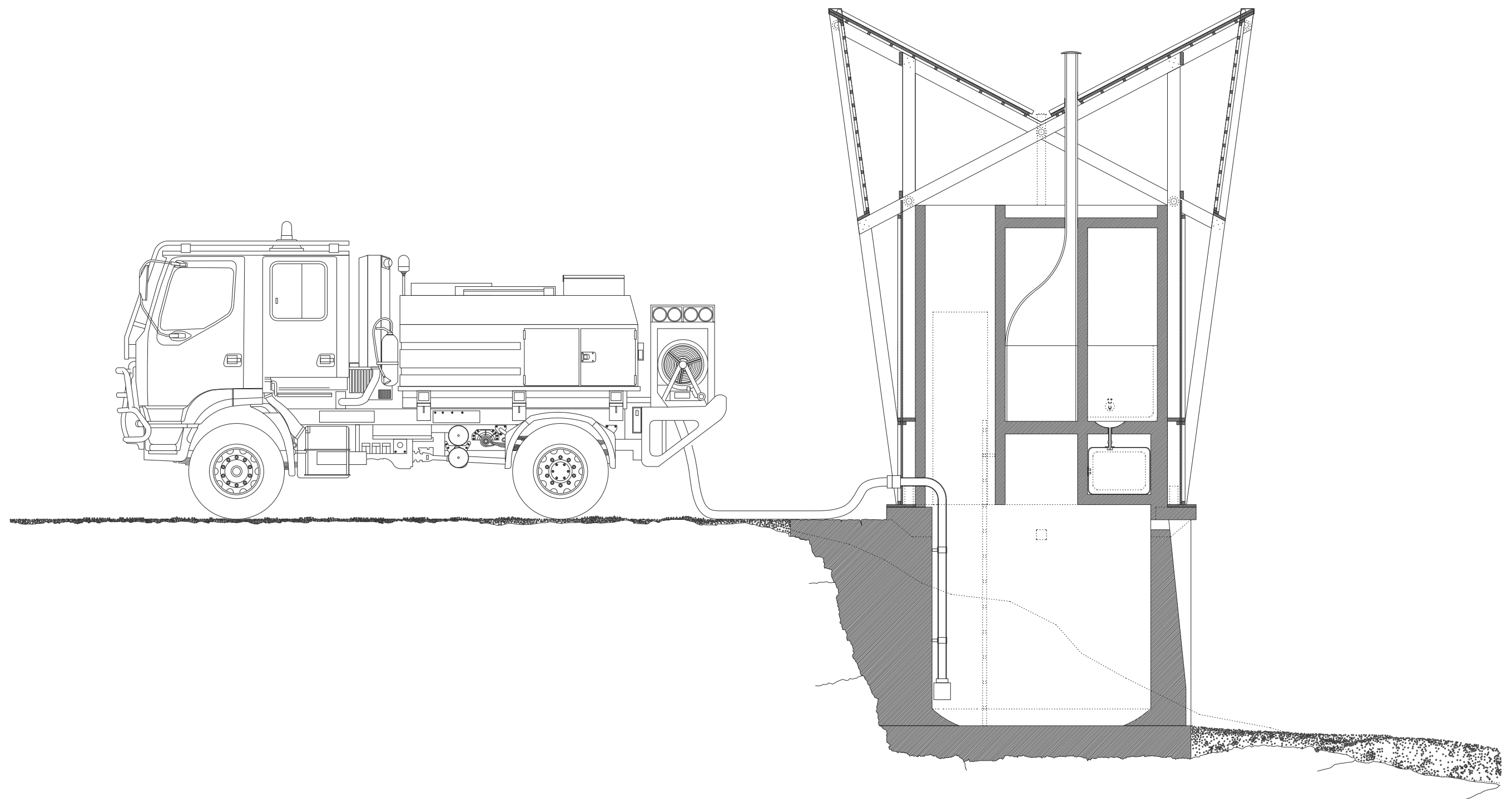
Coupe transversale BB' - échelle 1.50 -
