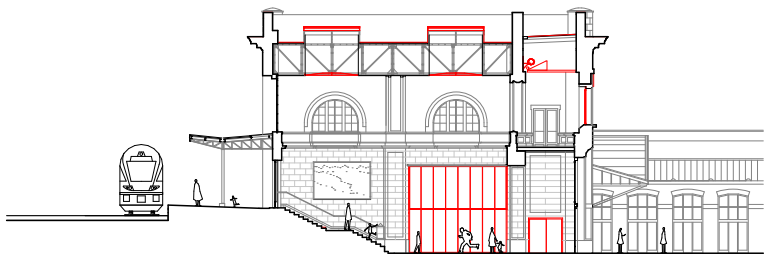
Coupe transversale 1:500
