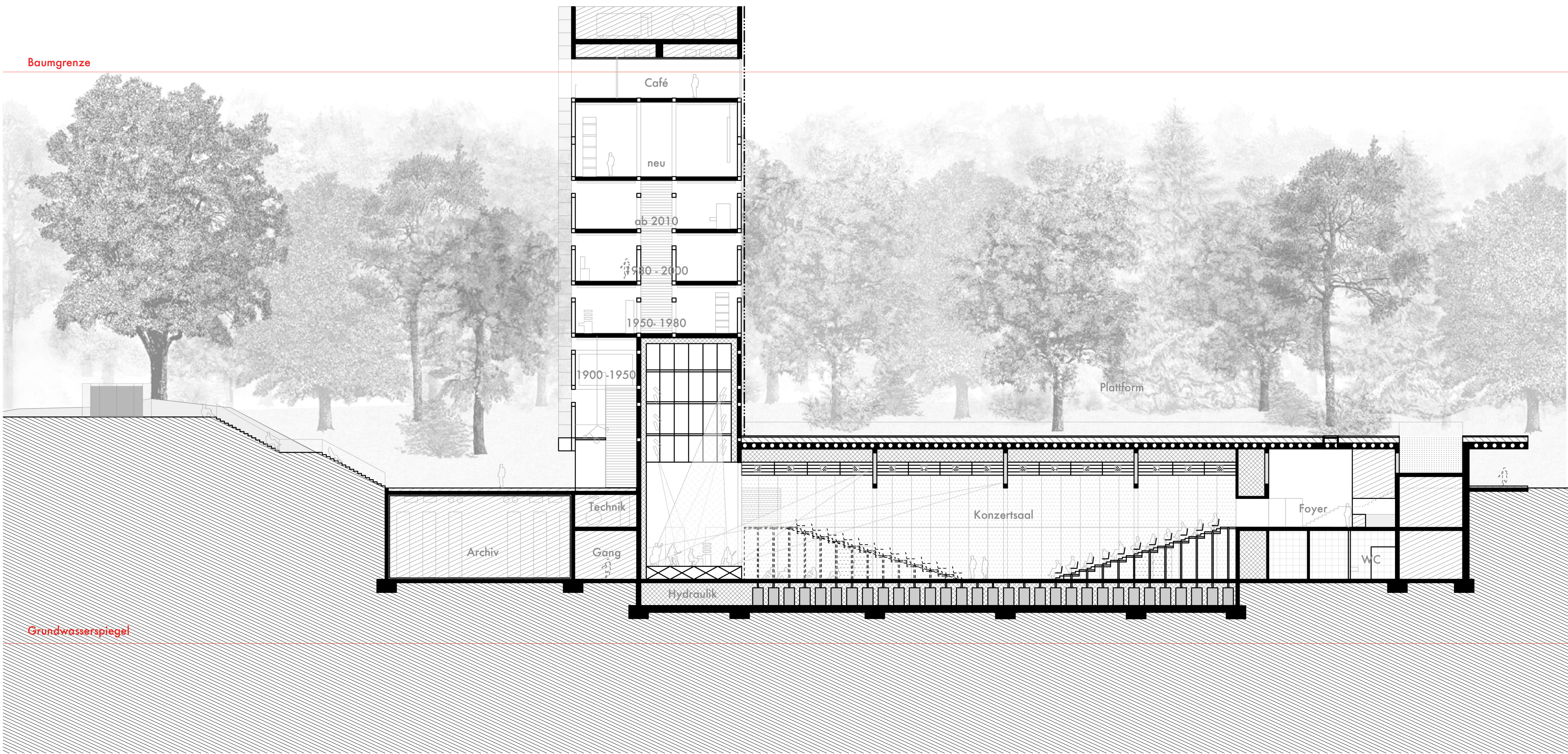
Schnitt aa
