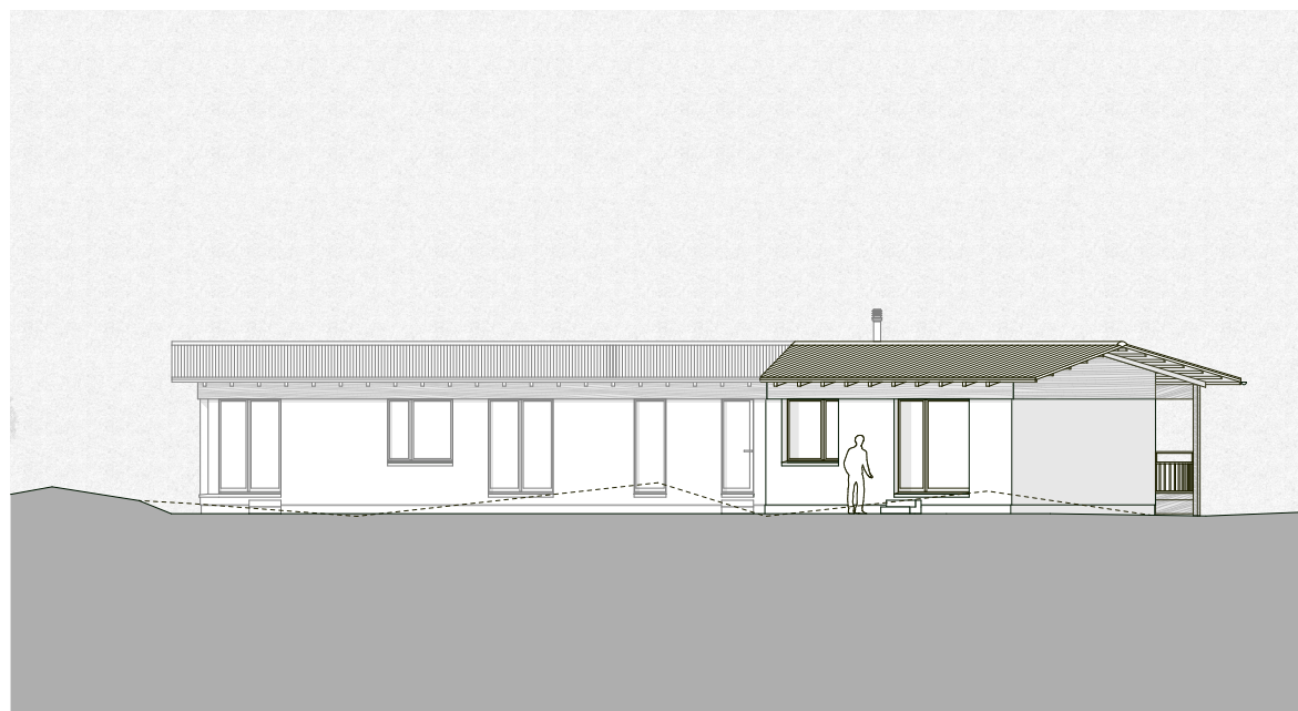
West- und Ostfassade 1:200
