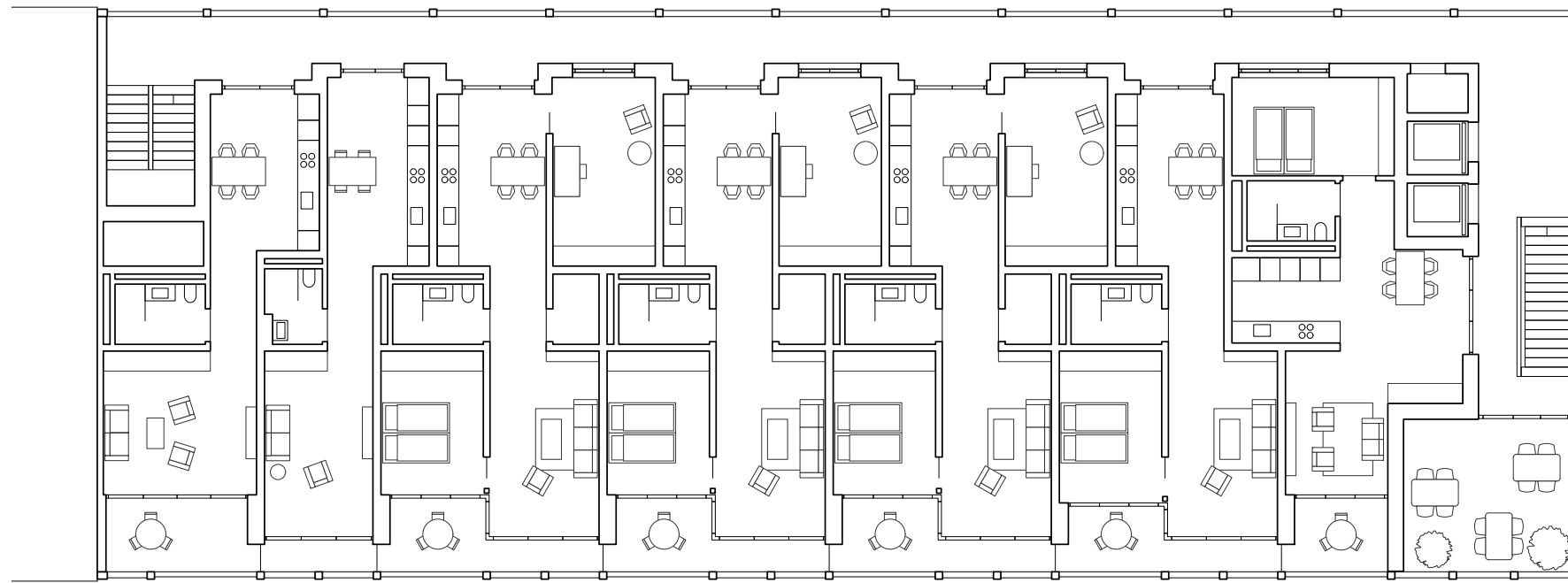
Grundriss 4. Obergeschoss Gemeinschaftsloggia 1:200
