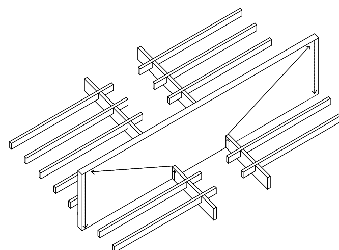
Die Wand zur Aula spannt von der Fassade zu Fassade und unterstützt die Längsträger der Doppelhalle um deren statische Höhe zu minimieren
