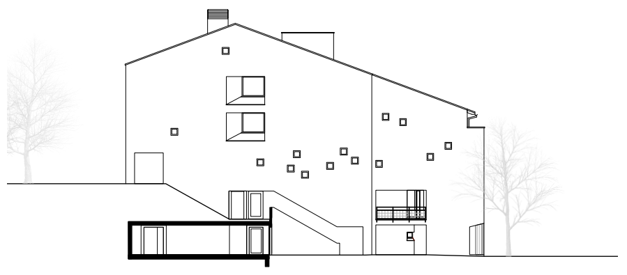
SÜDFASSADE 1:400
