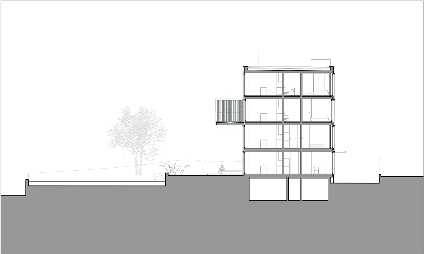
schnitt aa
