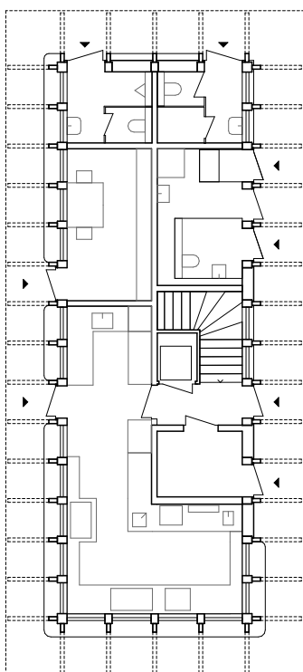
Erdgeschoss 1:200
