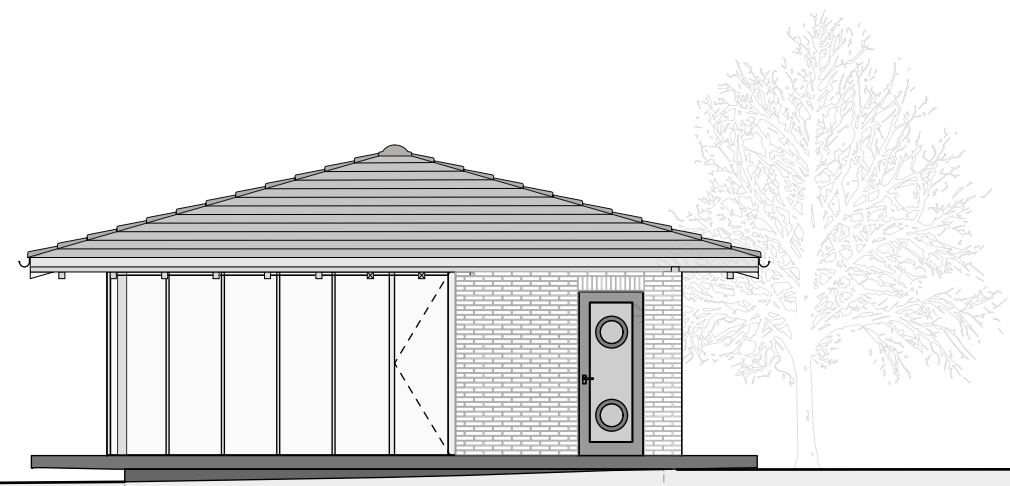
Nord-Ansicht
