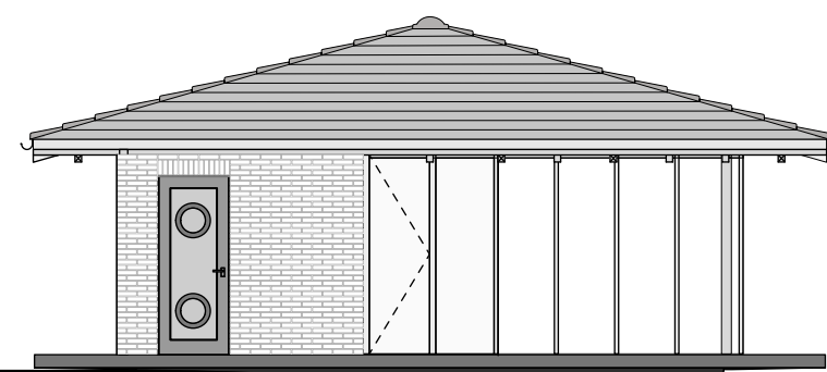
Süd-Ansicht
