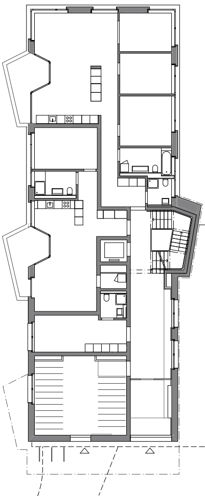
Erdgeschoss M 1: 400
