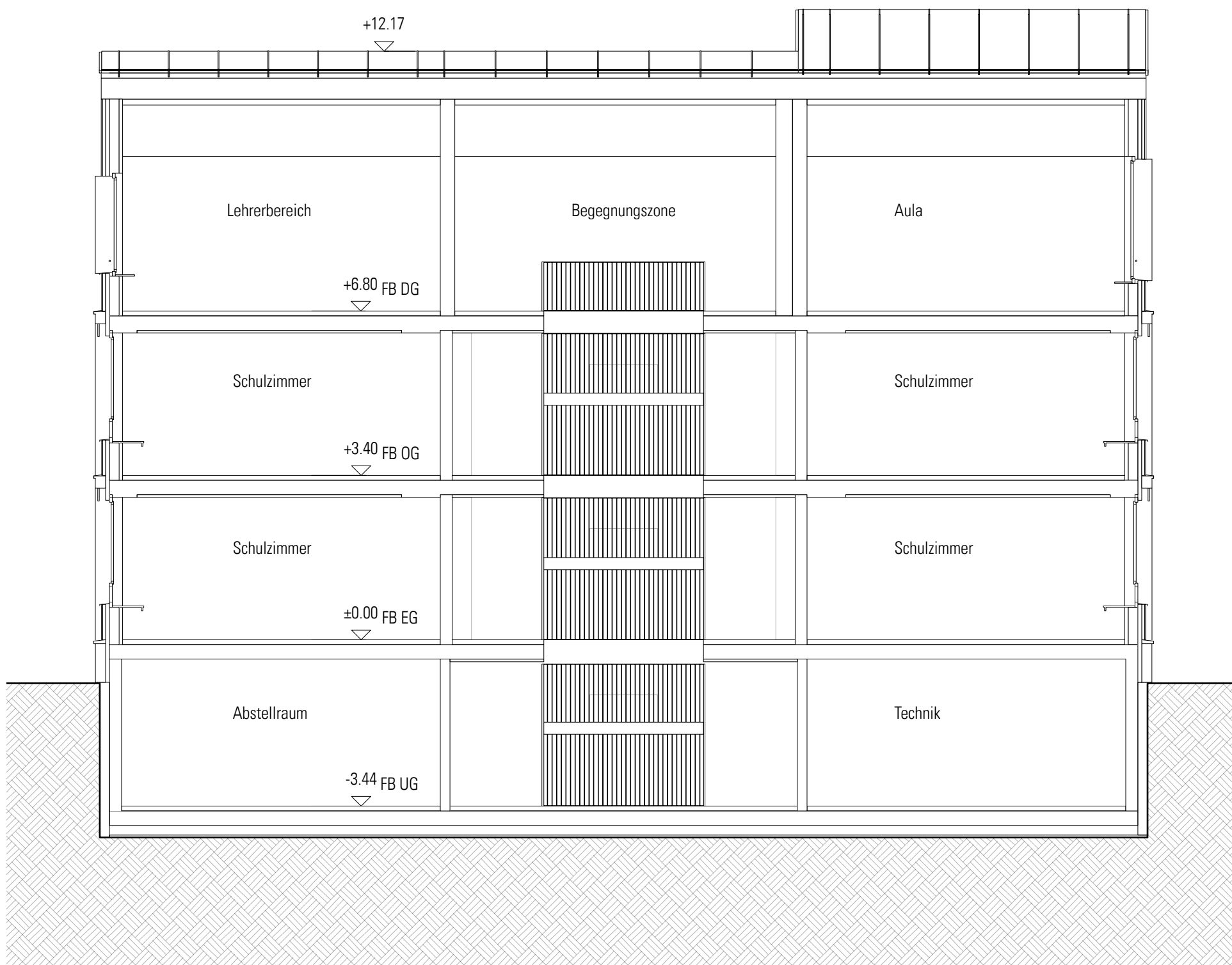
Schnitt DD
