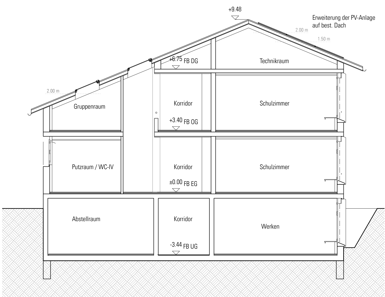
Schnitt BB
