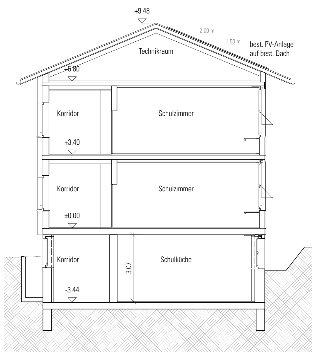
Schnitt AA
