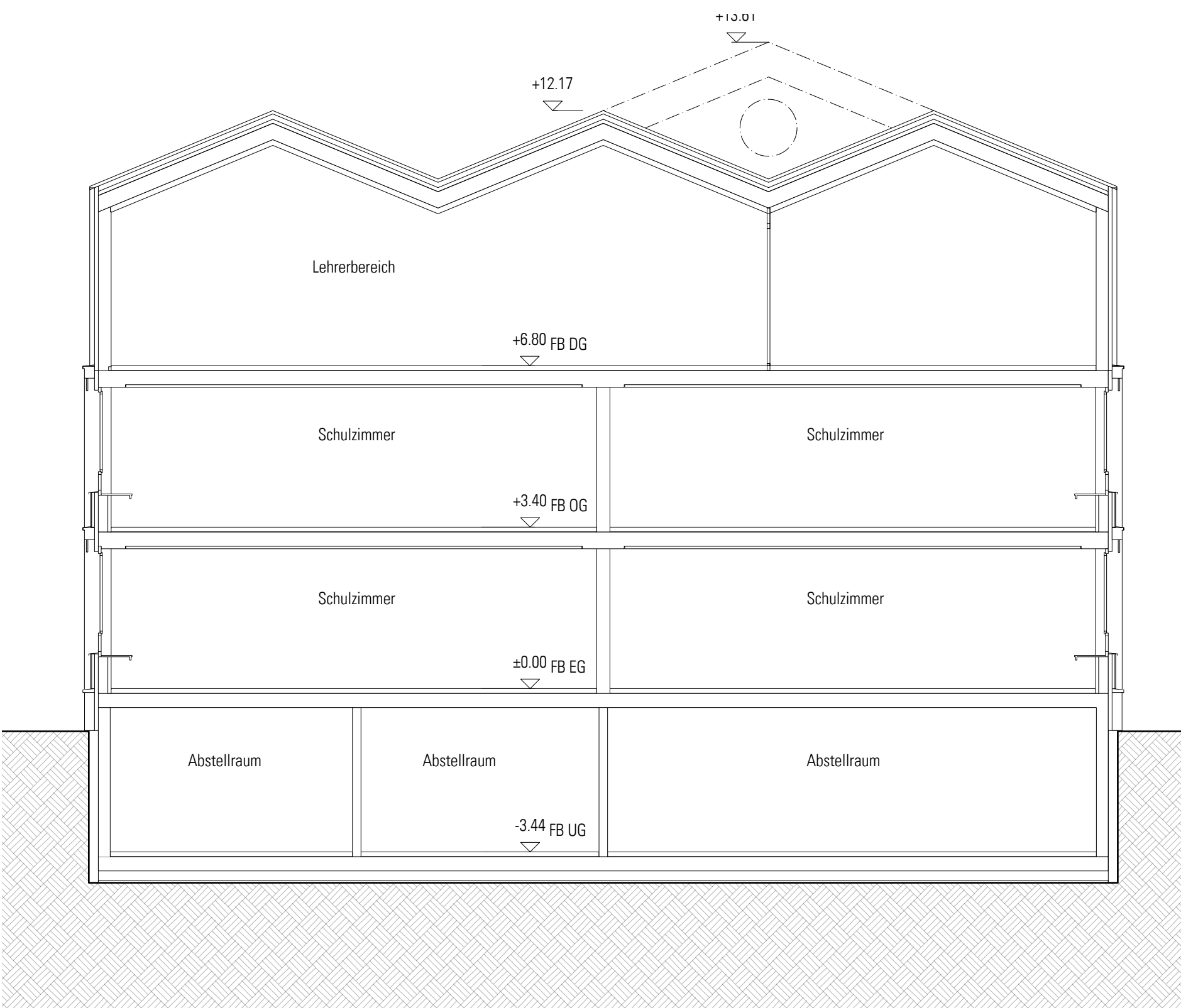
Schnitt CC
