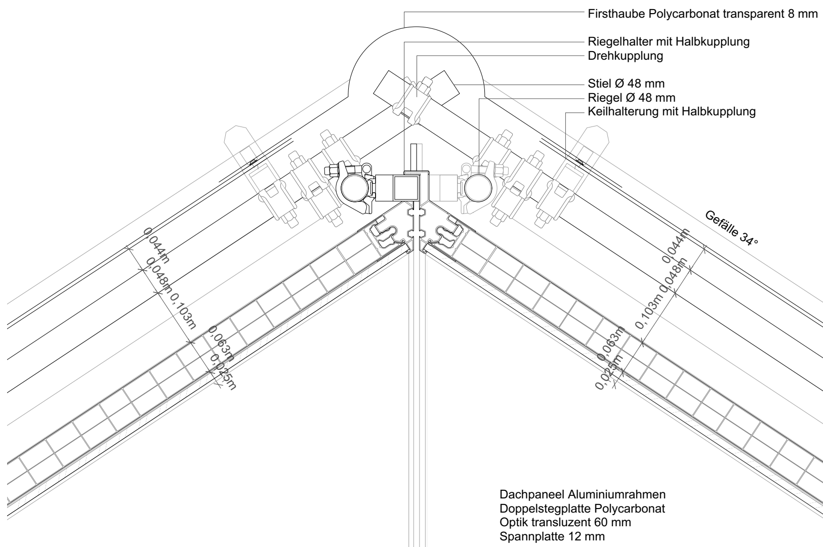
DETAIL SCHNITT FIRST
