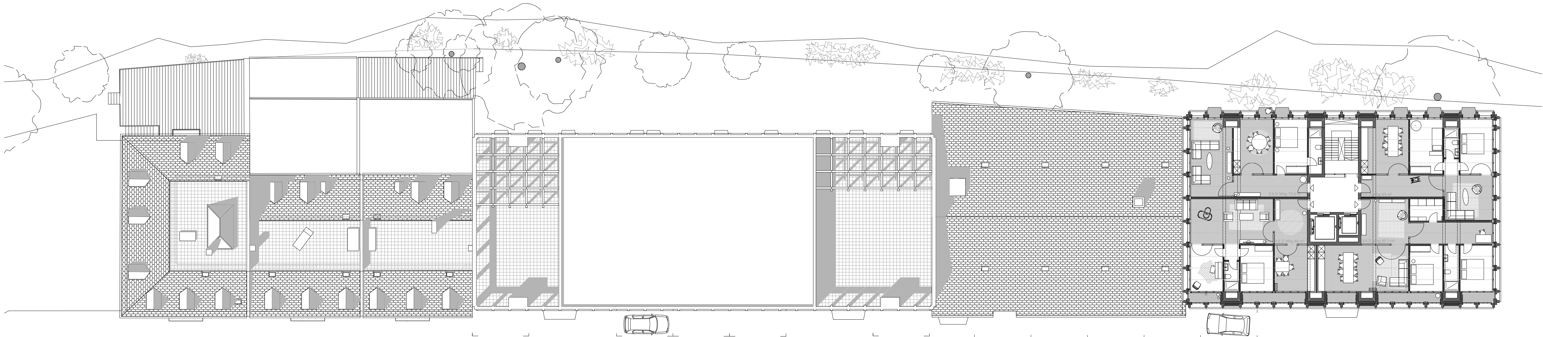
Dachaufsicht und Grundriss Wohnen 7. bis 12. OG 1:200
