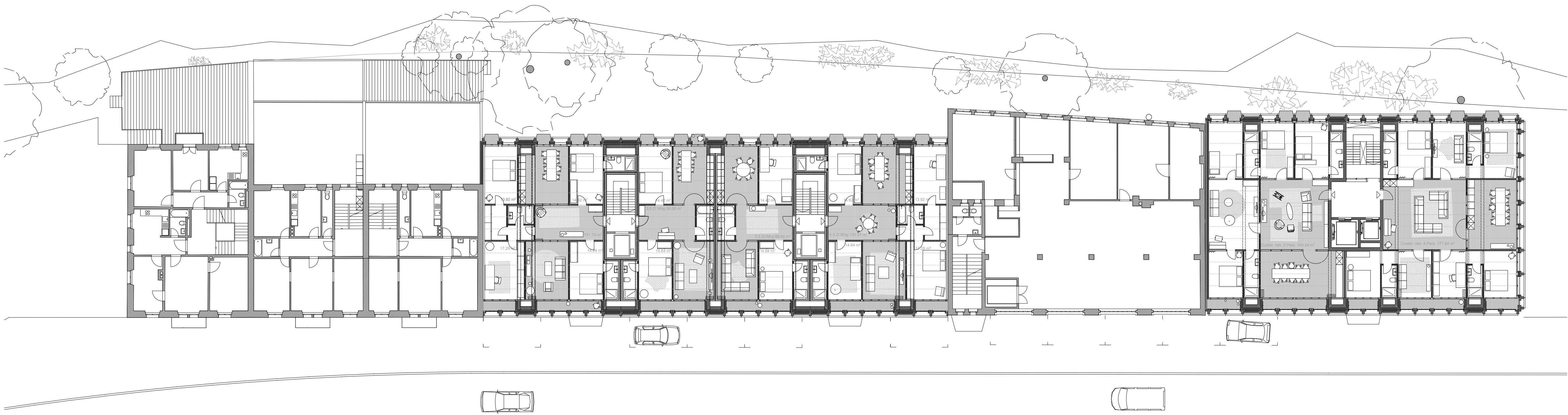
Grundriss Regelgeschoss Wohnen 1.-6. OG 1:200
