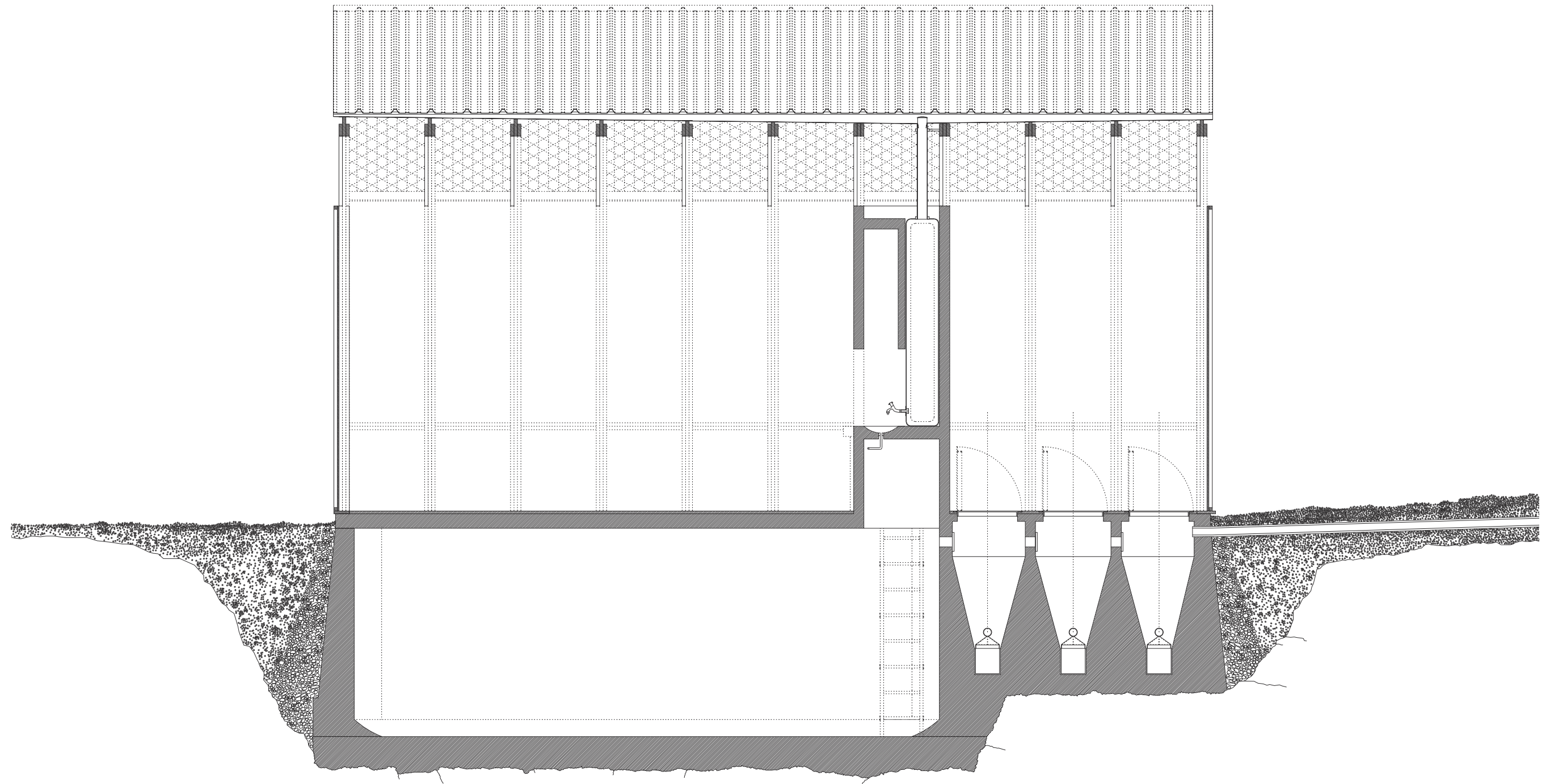
Coupe longitudinale - échelle 1.50 -
