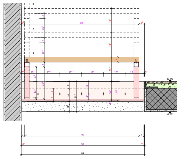
ANSICHT STIRNE - UNTEN
