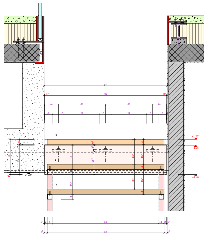
ANSICHT STIRNE - OBEN
