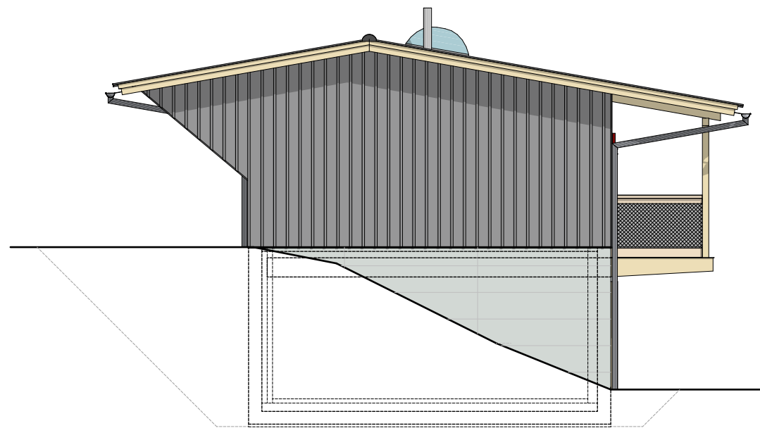
Südfassade
