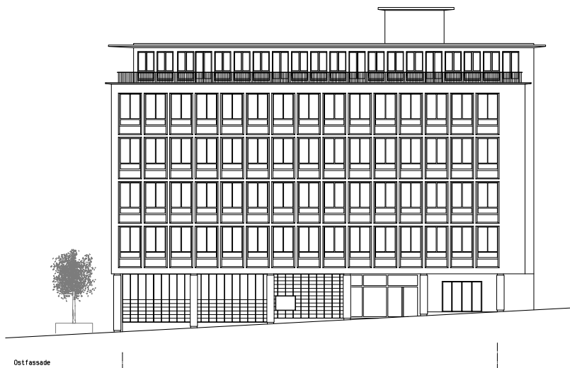
Ostfassade
