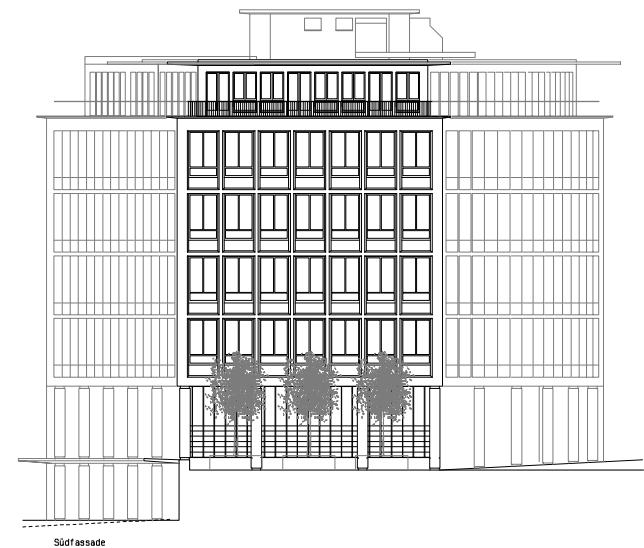
Südfassade
