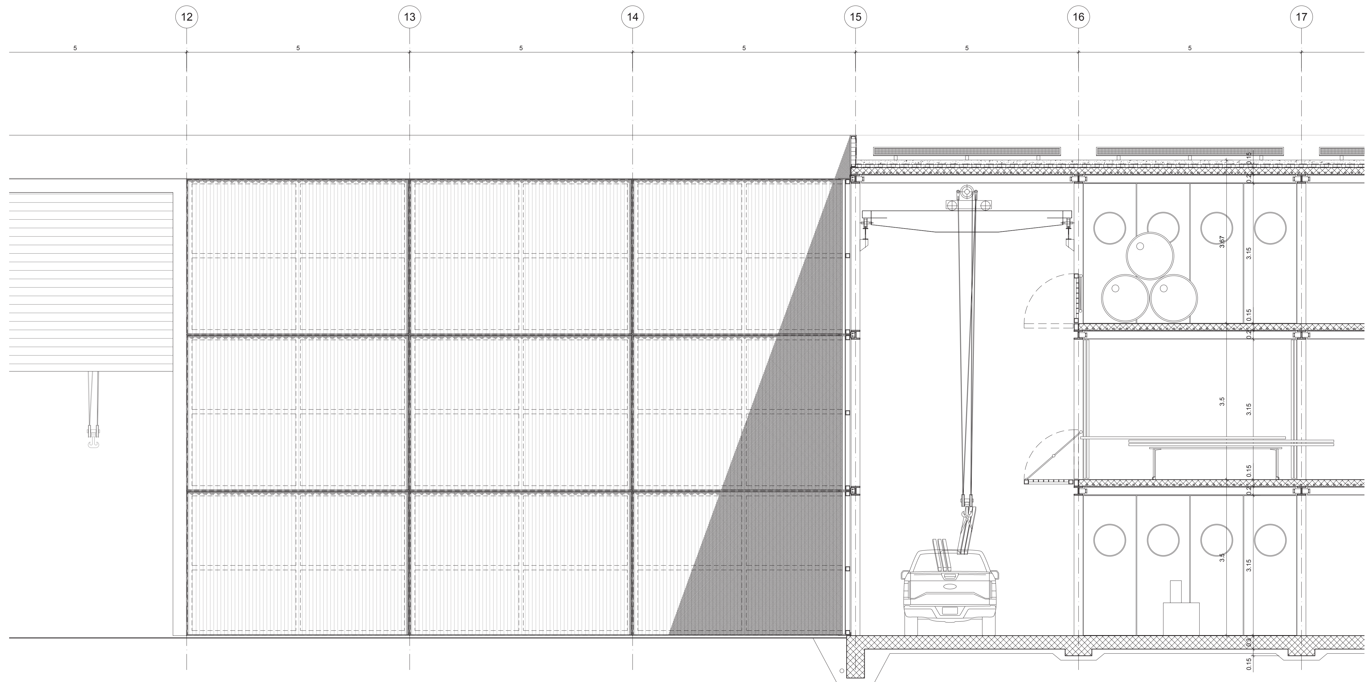
Coupe Longitudinale - Espace de chargement/ateliers Drive in, 1:50
