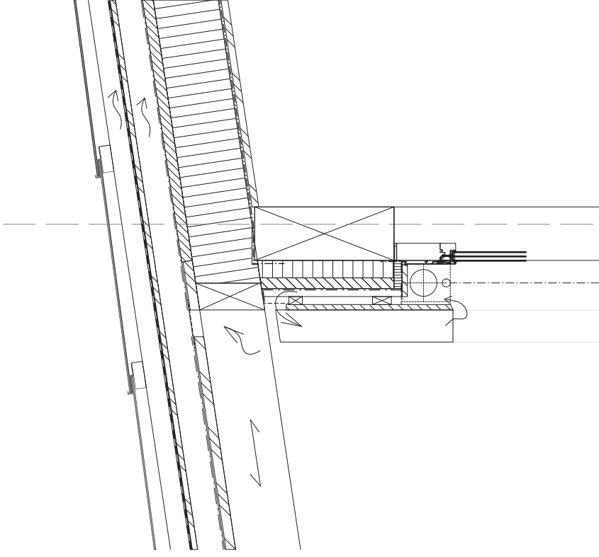
Dachanschluss
