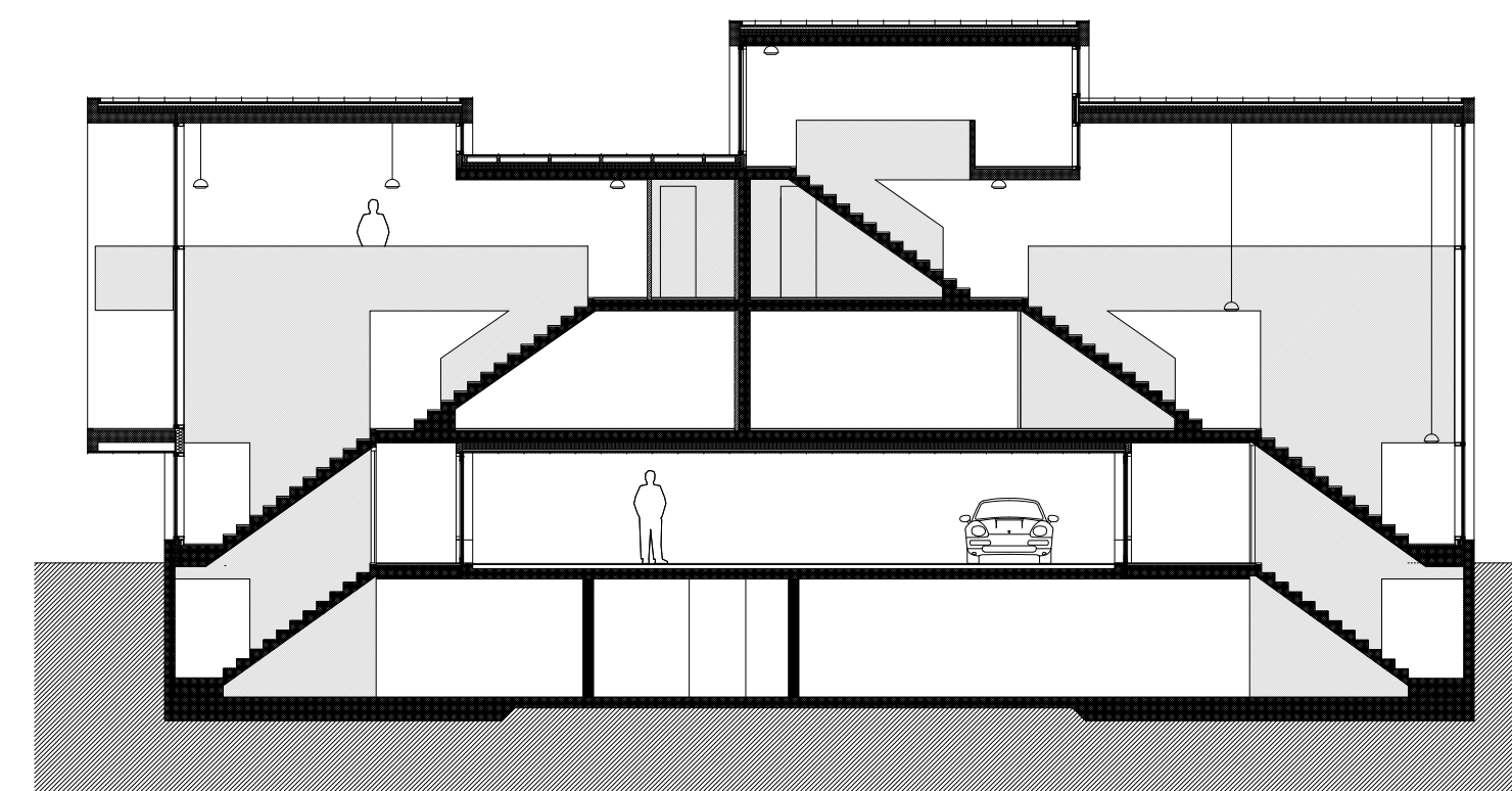
Schnitt
