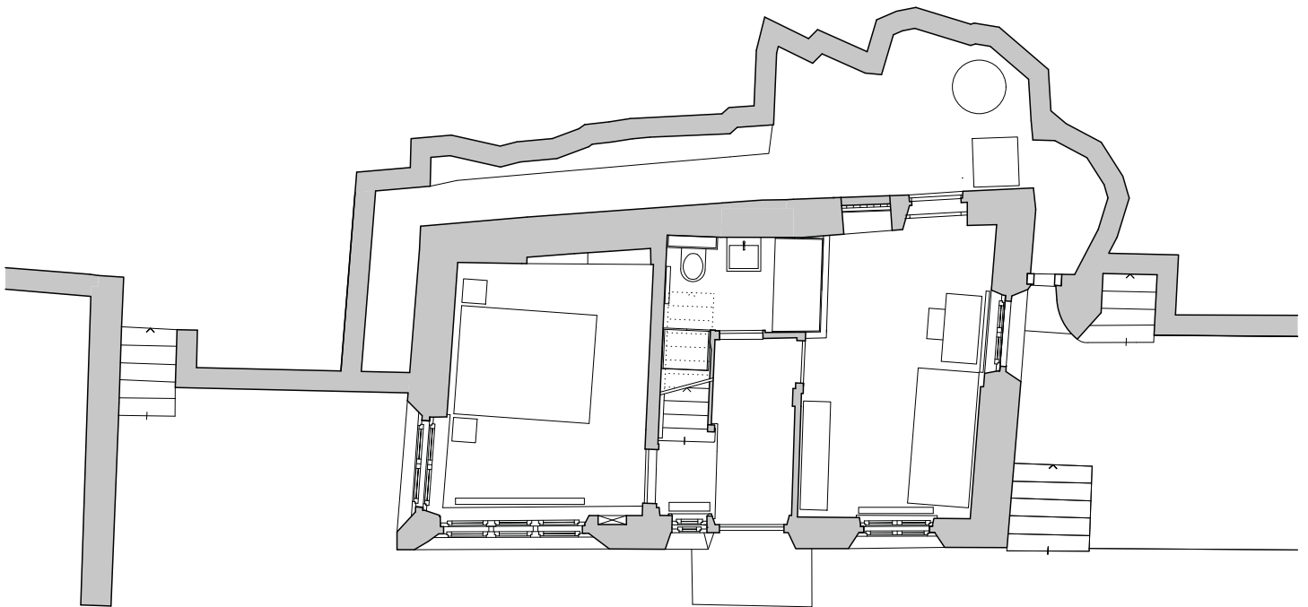
Grundriss Erdgeschoss
