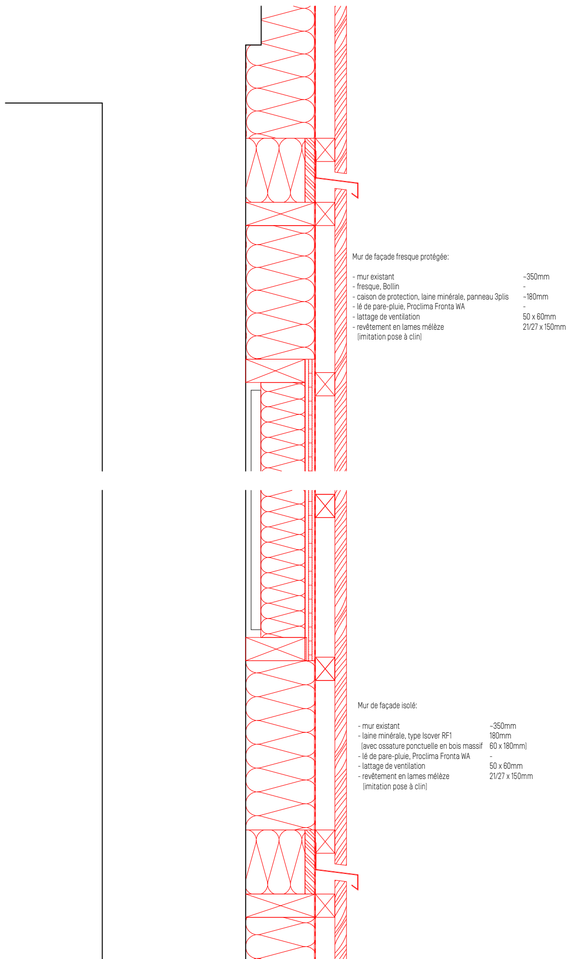
Détail en coupe 1:10, fresque recouverte sans l'endommager
