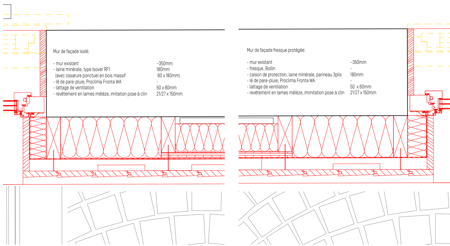
Détail en plan 1:10, fresque recouverte sans l'endommager
