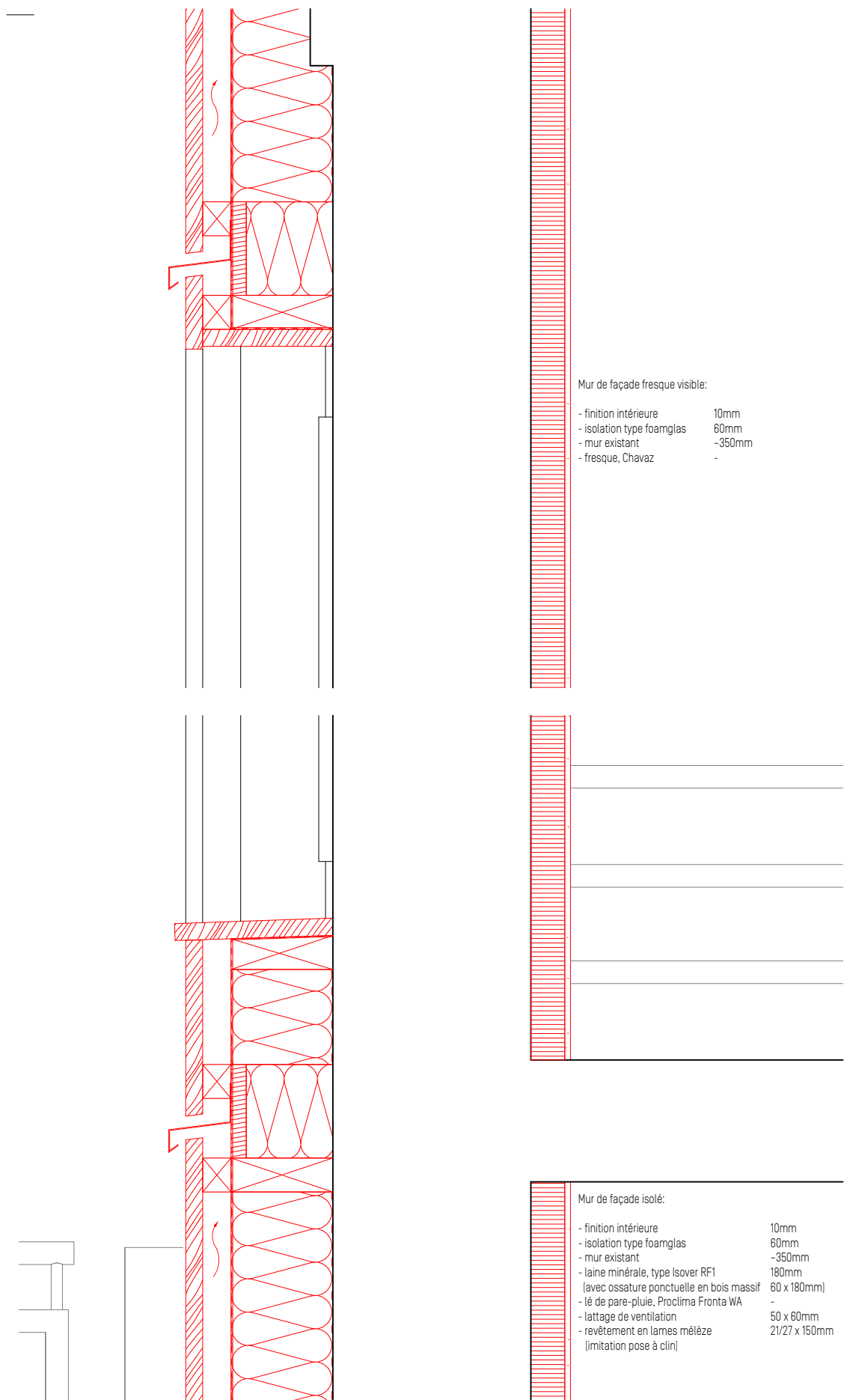
Détail coupe 1:10, fresque conservée visible
