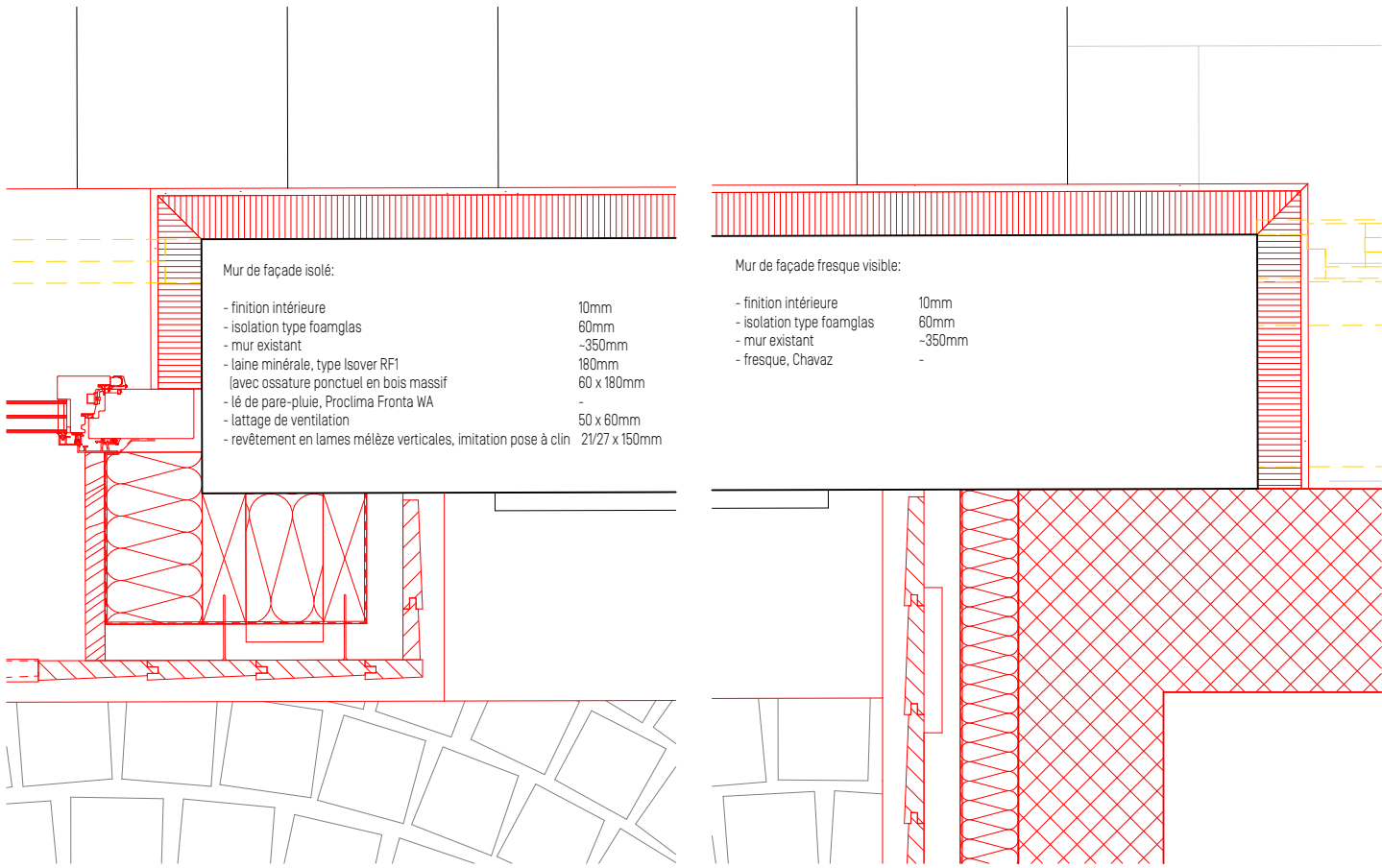
Détail en plan 1:10, fresque conservée visible
