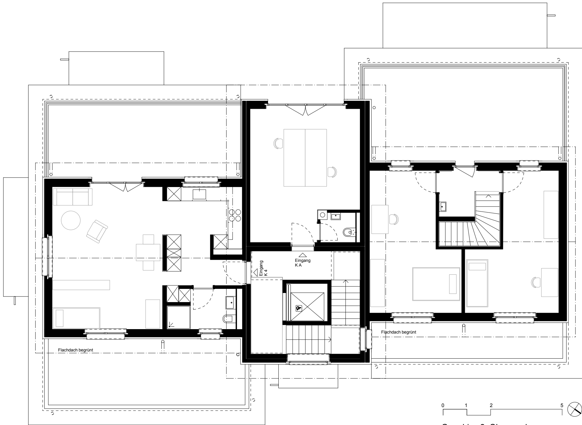
Grundriss 2. Obergeschoss
