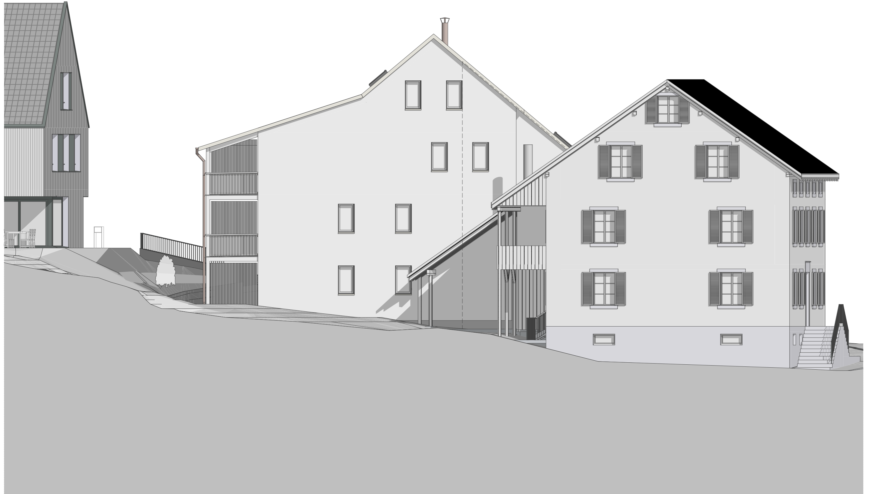
ANSICHT MFH SÜD / 1:100
